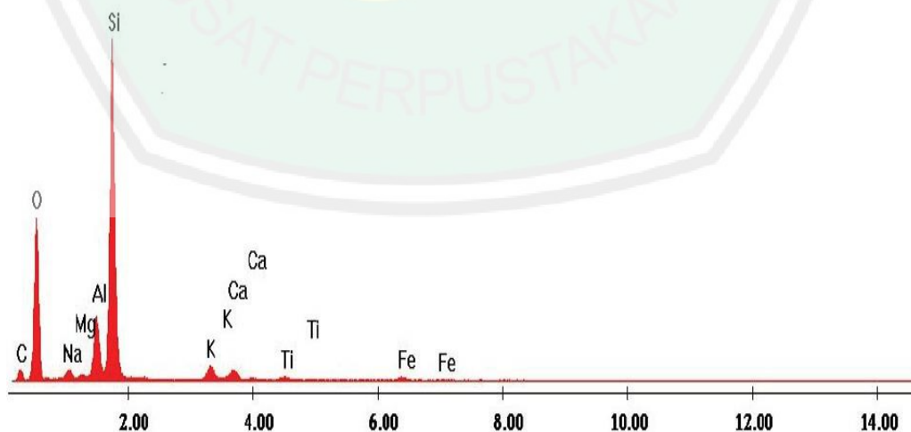
Gambar 2.12 Hasil analisis EDX pada Z-TiO 2 -SG (Ratiu, dkk., 2009)
