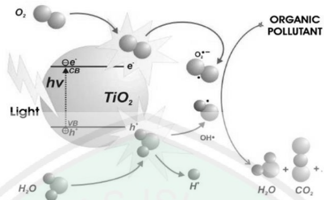
Gambar 2.6 Mekanisme reaksi fotokatalisis pada semikonduktor \text{TiO}_2 (Fujishima, dkk., 2008)
