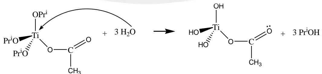
Gambar 4.1 Ilustrasi (1) mekanisme reaksi pelarutan menggunakan isopropanol; (2) Penambahan asam asetat; (3) Hidrolis menggunakan air (Leaustic, dkk., 1988; Fessenden dan Fessenden, 1986)
