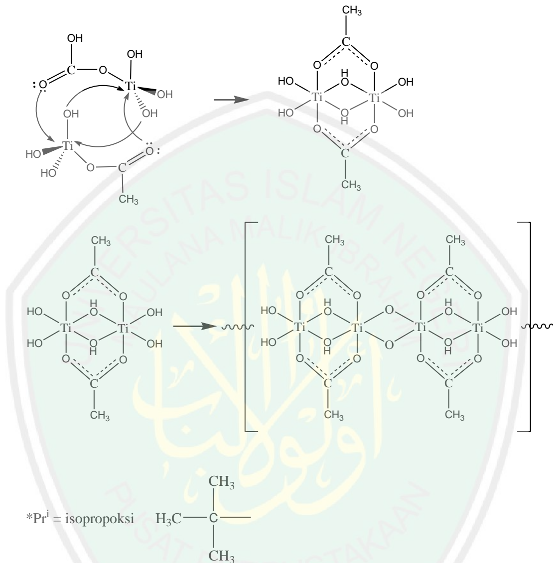
Gambar 4.2 Ilustrasi mekanisme reaksi pembentukan gel (polimerisasi) TiO 2 dengan metode sol-gel (Livage, dkk., 1988 ; Nolan, dkk., 2010 ; Brinker dan Scherer, 1990 ; Babounneau, dkk., 1988).
