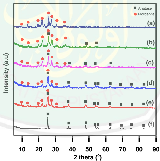
Gambar 4.7 Difraktogram : (a) zeolit mordenit (Chasanah, 2017); (b) \text{TiO}_2 /zeolit 5:95%; (c) \text{TiO}_2 /zeolit 10:90%; (d) \text{TiO}_2 /zeolit 20:80%; (e) \text{TiO}_2 /zeolit 30:70%; (f) \text{TiO}_2
