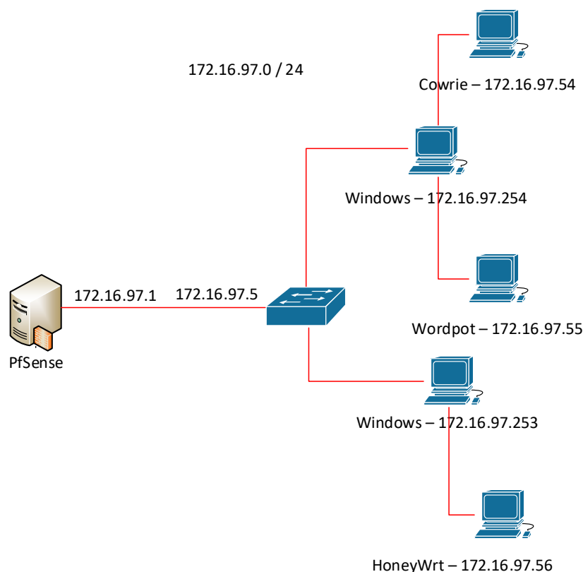
Figure 23 : Diagramme de la DMZ
