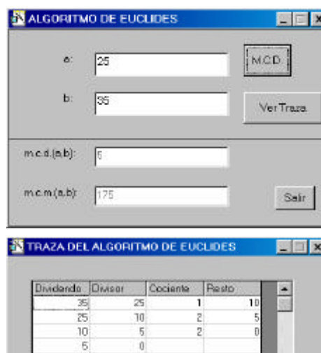
Figura 1. Algoritmo de Euclides
