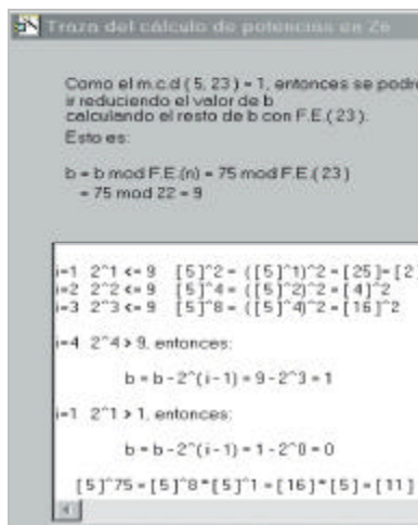
Figura 4. Cálculo de potencias en Z_n
