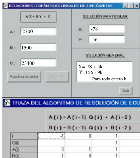
Figura 2. Ecuaciones diofánticas
