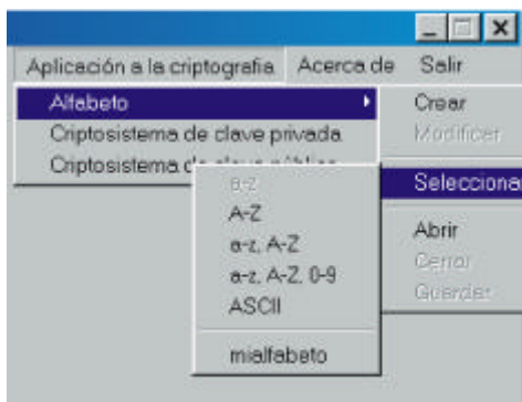
Figura 5. Elección del alfabeto
