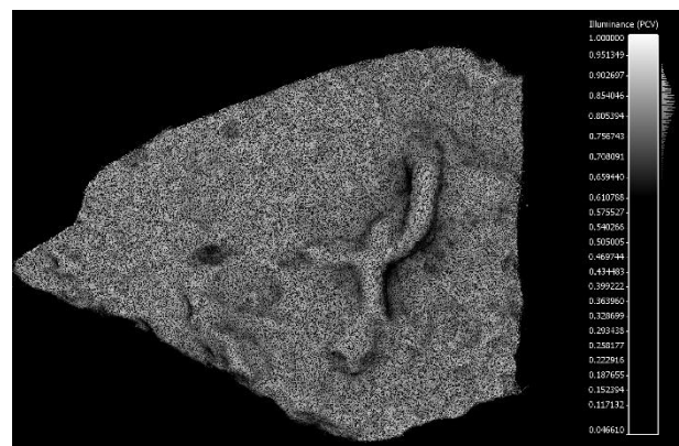
Figura 13: Técnica RTI sobre nube de puntos.
