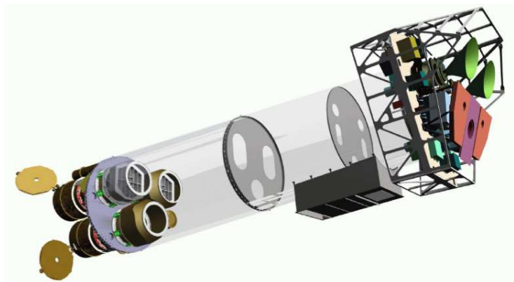
Figura 4.2. Esquema de los módulos contenidos a bordo del satélite XMM-Newton . Los módulos de espejos están equipados con los arreglos de redes de difracción ( Reflection Grating Arrays ) y se encuentran abajo a la izquierda. A la derecha se observan los instrumentos del plano focal: las cámaras EPIC MOS con sus radiadores (en negro y verde), el radiador de la cámara EPIC pn (en violeta), los detectores RGS (en celeste) y sus radiadores (en rosa). El telescopio OM está oscurecido por el módulo del espejo inferior. Imagen tomada de XMM-Newton Users Handbook .
