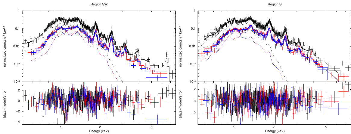
Figura 7.6. De izquierda a derecha, espectros de XMM-Newton de las cámaras PN y MOS1/2 correspondientes a las regiones SW y S, respectivamente. Las líneas sólidas indican el modelo del mejor ajuste (ver Tabla 7.2). Las líneas punteadas indican las contribuciones individuales de los modelos VAPEC y VNEI para cada cámara. El panel inferior muestra los residuos \chi^2 del ajuste..
