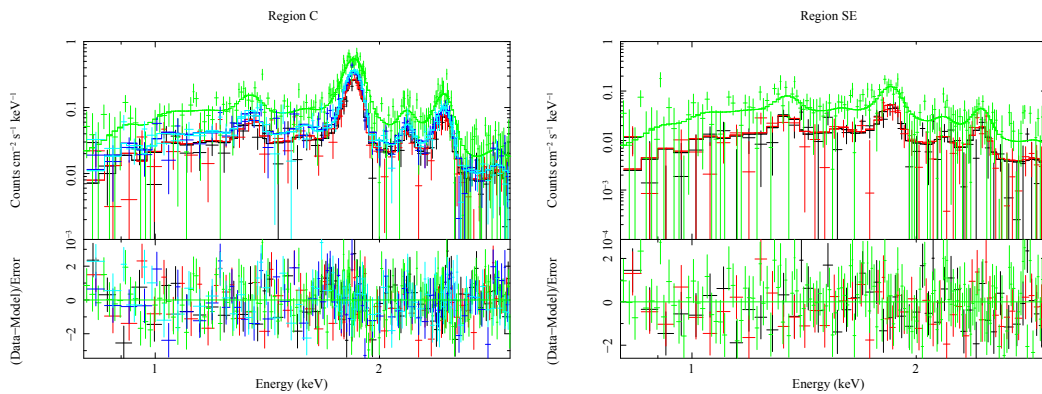
Figura 9.3. De izquierda a derecha: espectros de XMM-Newton correspondientes a las cámaras MOS1/2 y PN de las regiones C y SE, respectivamente. Las líneas sólidas indican el modelo del mejor ajuste (ver Tabla 9.2). Los paneles inferiores representan los residuos del ajuste \chi^2 .
