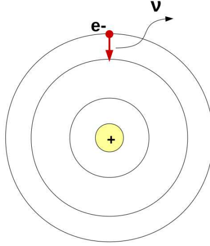
Figura 3.4. Esquema del proceso de emisión ligado-ligado. Este proceso se da a lugar cuando hay una transición directa entre dos estados ligados, pero prohibida de acuerdo a las reglas de selección.
