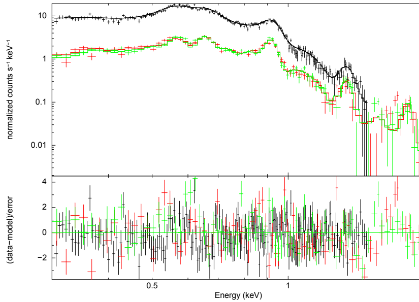
Figura 8.4. Espectros MOS1/2 y pn del fragmento G. Las líneas sólidas indican el modelo del mejor ajuste VNEI (ver Tabla 8.1). El panel inferior muestra los residuos del ajuste.
