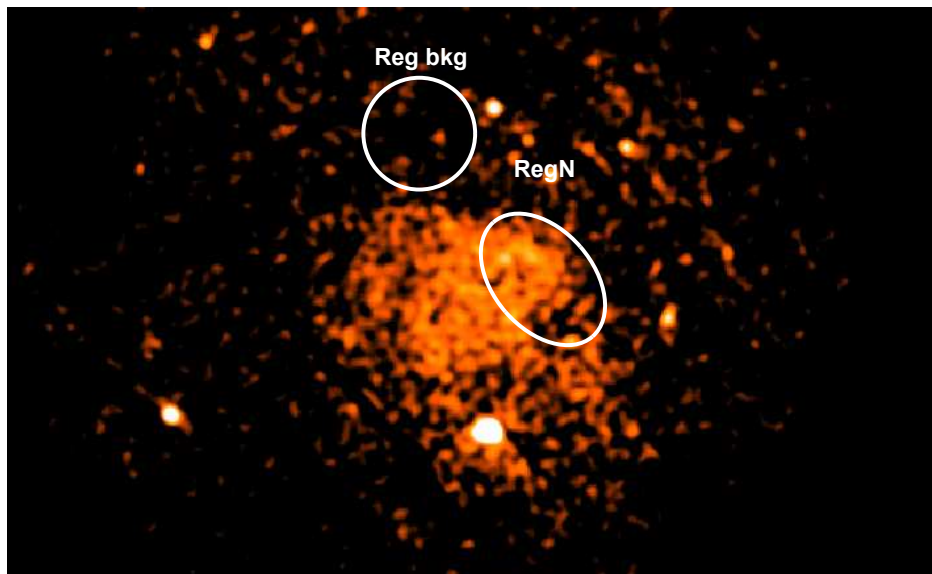
Figura 5.9. Regiones para extracción de espectro fuente (RegN) y fondo (Reg bkg) del RSN G309.2-0.6.
