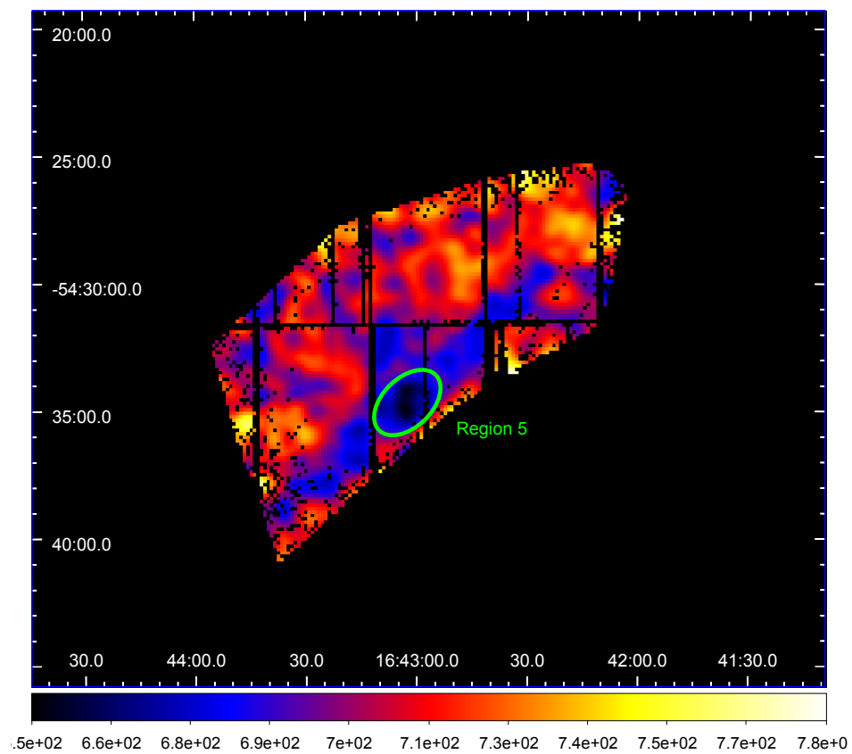
Figura 6.4. Mapa de energía media obtenido usando los datos de la cámara pn en el rango 0.5–1.0 keV (el tamaño del binnedo espacial es de 9 segundos de arco). Para los pixeles con menos de 8 cuentas se utilizó una máscara. La barra de color tiene una escala lineal, y el rango de energía indicado está entre 0.65 keV y 0.78 keV.
