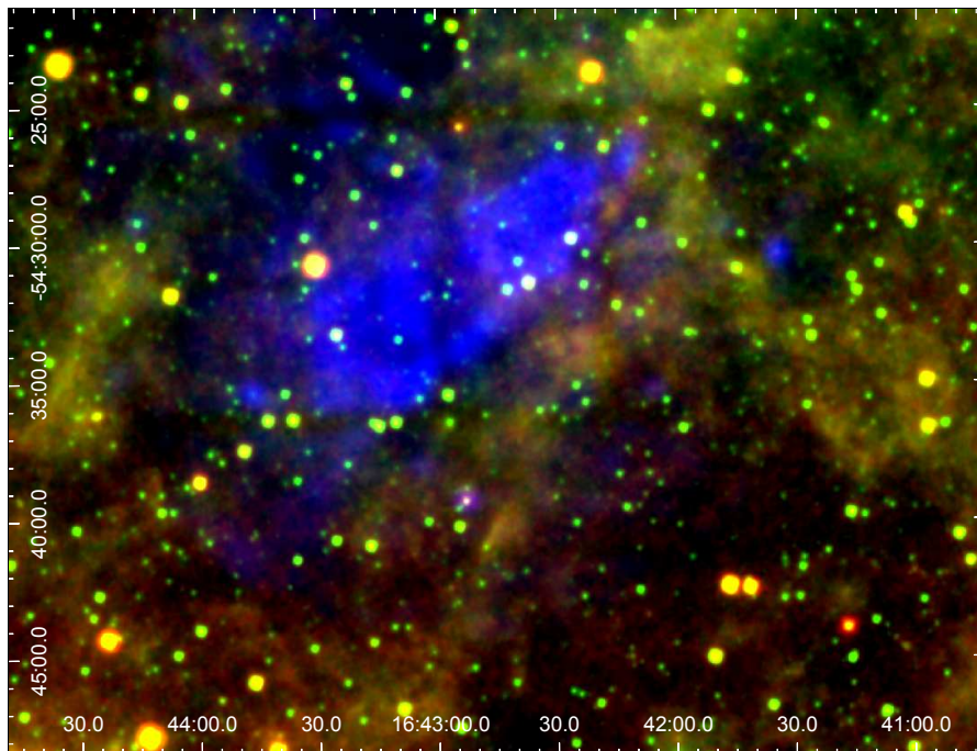
Figura 6.7. Se muestran en los colores verde y rojo observaciones en el infrarrojo de WISE en las bandas de 12 y 24 \mu\text{m} , respectivamente. En color azul se superpuso la emisión de rayos X blanda.
