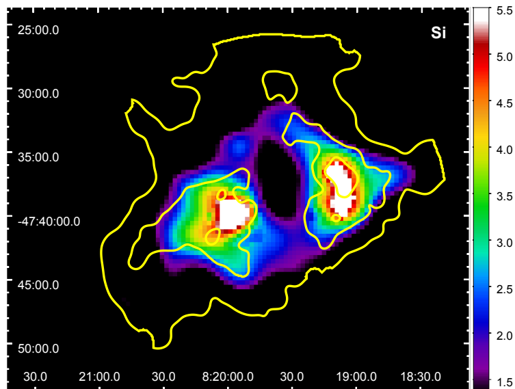
Figura 8.3. Mapa de cuentas en el rango de energía de 1.3–2.0 keV, correspondiente a la banda de Si, corregido por background y vignetting. Los contornos superpuestos en color amarillo representan la emisión en el rango de energía 0.3–3.0 keV. Los máximos de Si están espacialmente correlacionados con la emisión brillante en rayos X.
