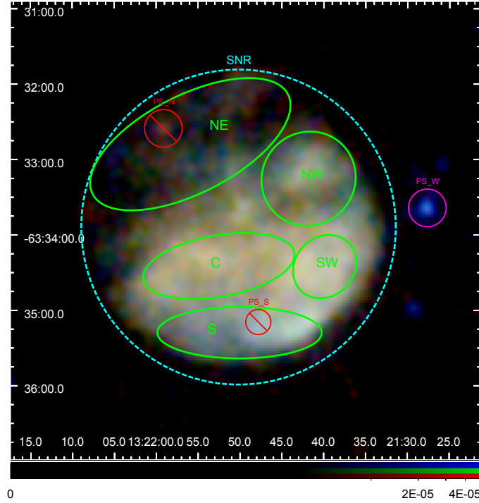
Figura 7.4. Imagen de XMM-Newton del RSN G306.3–0.9 en tres bandas de energía: en color rojo banda blanda de energía 0.5–1.0 keV, en color verde la banda media de energía 1.0–2.0 keV, en color azul banda dura de energía 2.0–4.5 keV. El contorno del RSN se indica en color cian y las regiones para las extracciones de espectros en color verde oscuro.
