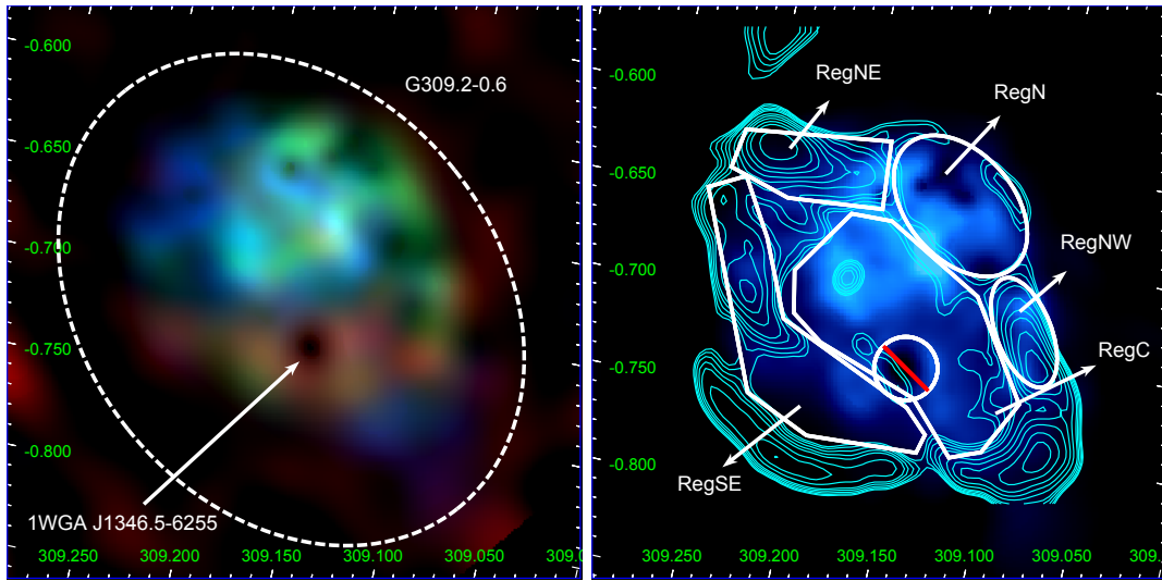
Figura 9.1. Izquierda: Mosaico de G309.2–0.6 en tres bandas de energía de rayos X: en color rojo el rango 0.3–1.2 keV, en color verde el rango 1.2–2.0 keV y en color azul en el rango 2.0–3.0 keV. Derecha: Mosaico en el rango de energía de rayos X de 0.8–3.0 keV, superpuesto con contornos de radio a 843 MHz indicados en color cian. En color blanco se indican las regiones para el análisis espectral. Ambas imágenes fueron corregidas por contaminación de fondo, exposición y vignetting.
