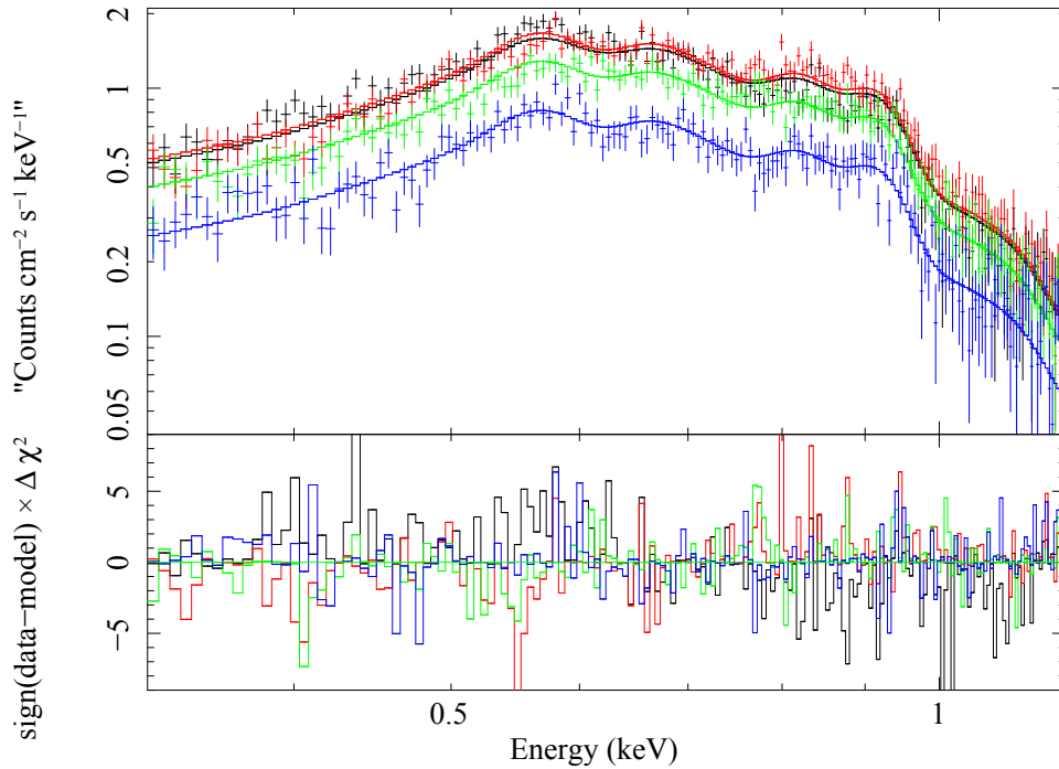
Figura 6.5. Espectro de rayos X de G332.5– 5.6 obtenido a partir de los datos de la cámara pn. Los colores indican las diferentes regiones: Región 1 en color negro, Región 2 en color rojo, Región 3 en color verde y Región 4 en color azul. Las líneas solidas indican el modelo del mejor ajuste (ver Tabla 6.1). El panel inferior muestra los residuos del ajuste \chi^2 .
