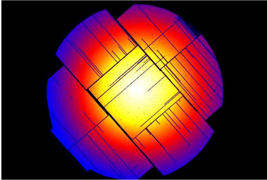
Figura 5.3. Mapa de exposición para la observación del RSN G309.2-0.6 en el rango de energía 0.5 a 10 keV, construido a partir de la lista de eventos filtrada de la cámara EPIC MOS1.
