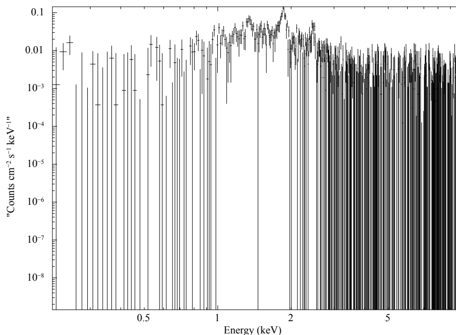
Figura 5.10. Espectro de la RegN del RSN G309.2-0.6 con el fondo (Reg bkg) sustraído, el cual fue extraído de los datos correspondientes a la cámara MOS1.
