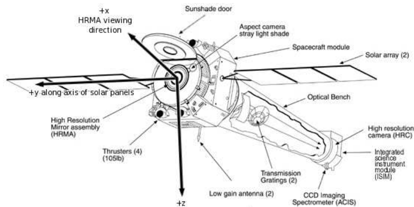
Figura 4.6. Esquema de la carga a bordo del Observatorio Chandra . Imagen tomada de The Chandra Proposers' Observatory Guide .
