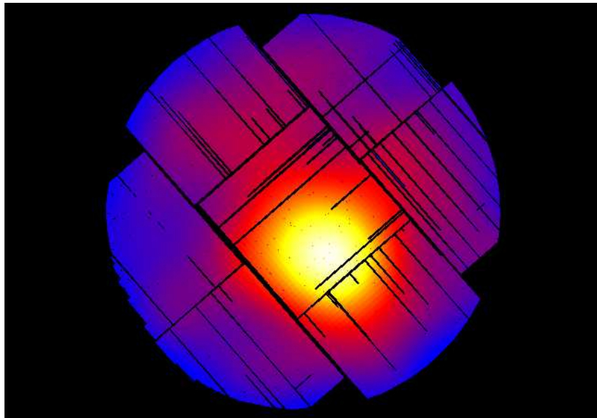
Figura 5.5. Fondo para la cámara EPIC MOS1, realizada a partir del enmascarado de las fuentes puntuales resultantes de la tarea eboxdetect.
