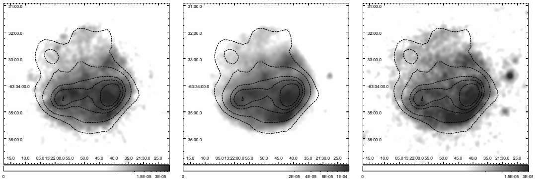
Figura 7.1. Imágenes de rayos X del RSN G306.3–0.9, observados por XMM-Newton, en tres bandas de energía. Izquierda: rango blando de energía 0.5–1.0 keV. Medio: rango medio de energía 1.0–2.0 keV. Derecha: rango duro de energía 2.0–4.5 keV. Las imágenes se suavizaron con una función Gaussiana 2-D con un kernel de \sigma = 20 segundos de arco. Los contornos superpuestos corresponden a datos en la frecuencia de radio de 843 MHz, en los niveles 2, 4, 10, 12 y 19 mJy beam -1 , los cuales fueron tomados del catálogo MOST Supernova Remnant Catalog (Whiteoak & Green, 1996).
