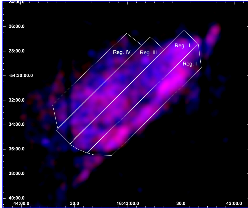
Figura 6.2. Imagen de la emisión en rayos X blandos obtenida por la cámara MOS2 de la región central del RSN G332.5–5.6. Los rangos de energía 0.3–0.6 keV y 0.6–1.0 keV están indicados en los colores rojo y azul, respectivamente. Las regiones utilizadas en el análisis espectral están indicadas en color blanco. En esta imagen el norte es hacia arriba y el este hacia la izquierda.
