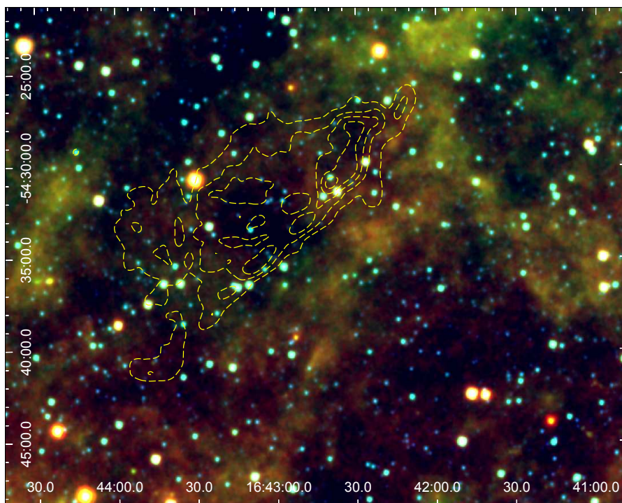
Figura 6.8. En la imagen se representan observaciones de WISE en las bandas de 4.6, 12 y 24 \mu\text{m} en los colores azul, verde y rojo, respectivamente, y superpuestos, en color amarillo, se pueden ver los contornos de emisión X blanda correspondientes al remanente.
