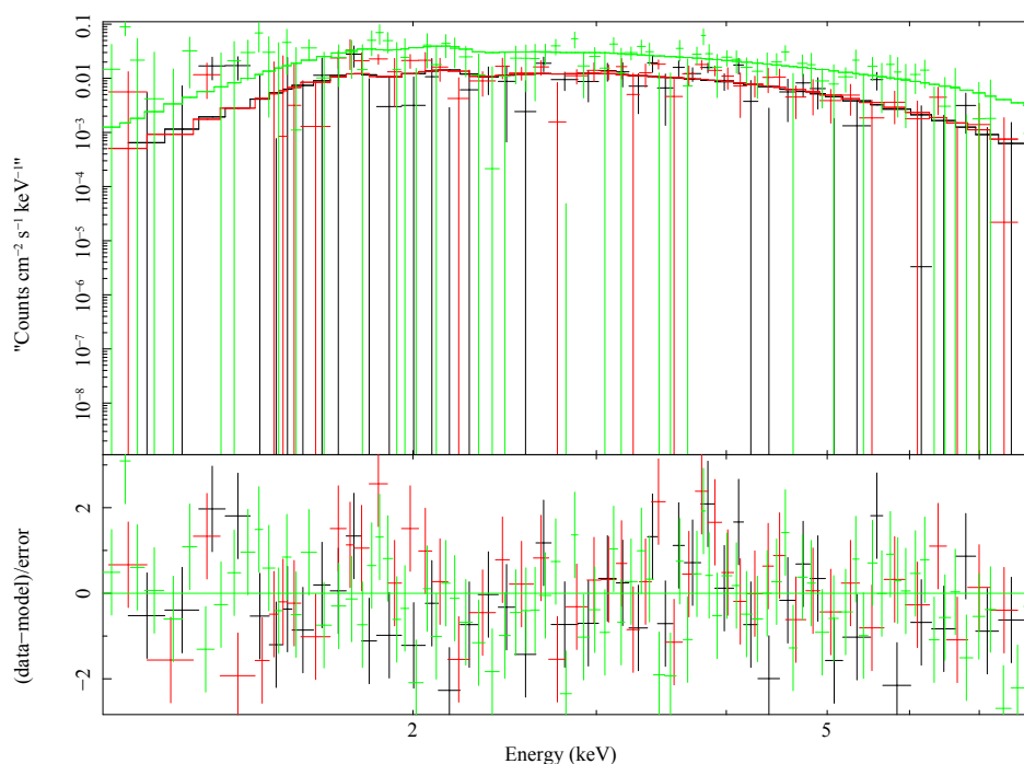
Figura 3.5. Espectro de origen no térmico correspondiente al RSN G32.4–0.1.
