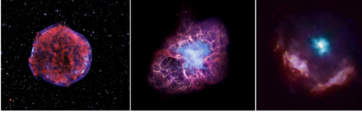
Figura 2.5. Izquierda: RSN Tycho, de tipo cáscara visto en longitudes de rayos X y óptico. La paleta de colores por energías es la siguiente: 1.6-2.15 keV en color rojo, 7.15-9.3 keV en color verde, 4-6 keV en color azul. Crédito: rayos X, NASA/CXC/Rutgers/K.Eriksen et al.; óptico DSS. Fuente: Chandra Image Gallery. Medio: RSN Crab Nebula, de tipo plerión. Se puede ver en color azul la emisión de rayos X, en los colores rojo y amarillo la emisión óptica y en color violeta la emisión infrarroja. Crédito: rayos X NASA/CXC/SAO/F.Seward; óptico NASA/ESA/ASU/J.Hester & A.Loll; infrarrojo NASA/JPL-Caltech/Univ. Minn./R.Gehrz. Fuente: Chandra Image Gallery. Derecha: RSN KES 75, de tipo compuesto. En color rojo/verde se pueden ver rayos X blandos, y en color azul rayos X duros. Crédito: NASA/CXC/GSFC/F.P.Gavriil et al. Fuente: Chandra Image Gallery.
