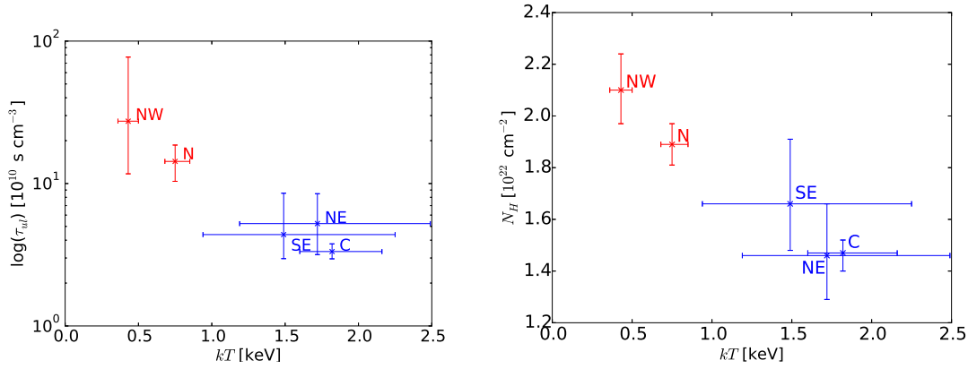
Figura 9.4. Izquierda: temperaturas vs escalas temporales de ionización \tau_{ul} para las cinco regiones seleccionadas. Derecha: valores de temperatura y densidad columnar N_H para las cinco regiones. En ambos paneles, el color azul indica valores bajos de \tau_{ul} , y valores altos de kT y de N_H , mientras que el color rojo indica valores altos de \tau_{ul} , y valores bajos de kT y de N_H .
