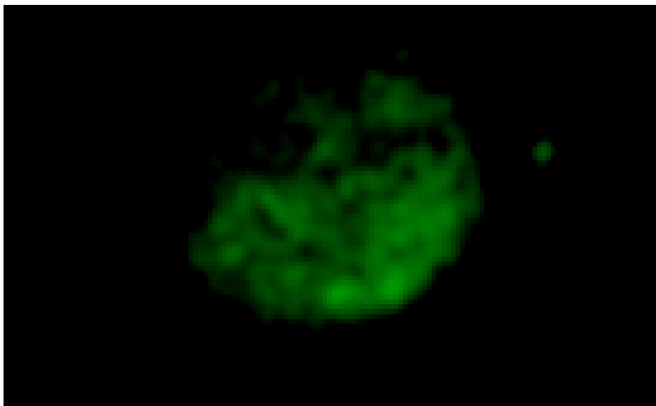
Figura 5.1. Mosaico del RSN G306.3-0.9 en el rango de energía 2100 a 2800 keV, correspondientes a la banda de S, construido a partir de los datos EPIC MOS1/2.
