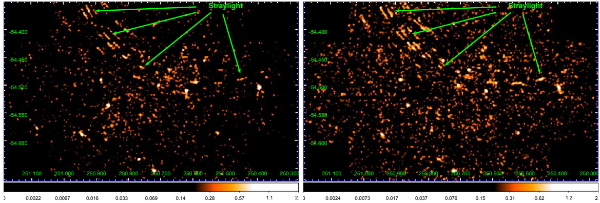
Figura 6.3. Imágenes de la cámara MOS2 del campo del RSN G332.5–5.6 donde puede observarse contaminación straylight y ausencia de emisión del remanente. Izquierda: rango de energía medio de 1.2 a 2 keV Derecha: rango de energía duro de 2.0 a 10 keV.
