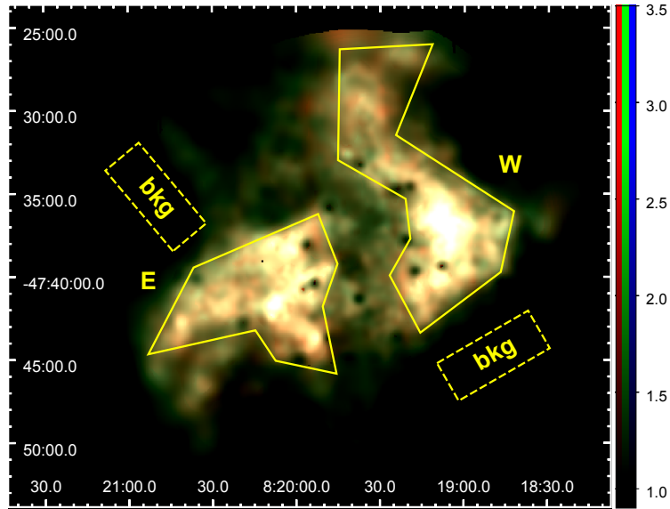
Figura 8.2. Imagen del fragmento G de Vela obtenida a partir de los datos de XMM-Newton. En color rojo se representa la banda de energía entre 0.3–0.6 keV, en verde la banda 0.6–1.3 keV y en color azul la banda 1.3–3.0 keV. Los contornos superpuestos en color amarillo representan las regiones de extracción de espectros este (E) y oeste (W). Los rectángulos punteados son las regiones elegidas para la extracción de espectros de fondo (bkg). Esta imagen fue corregida por background, vignetting, y las fuentes puntuales fueron removidas.
