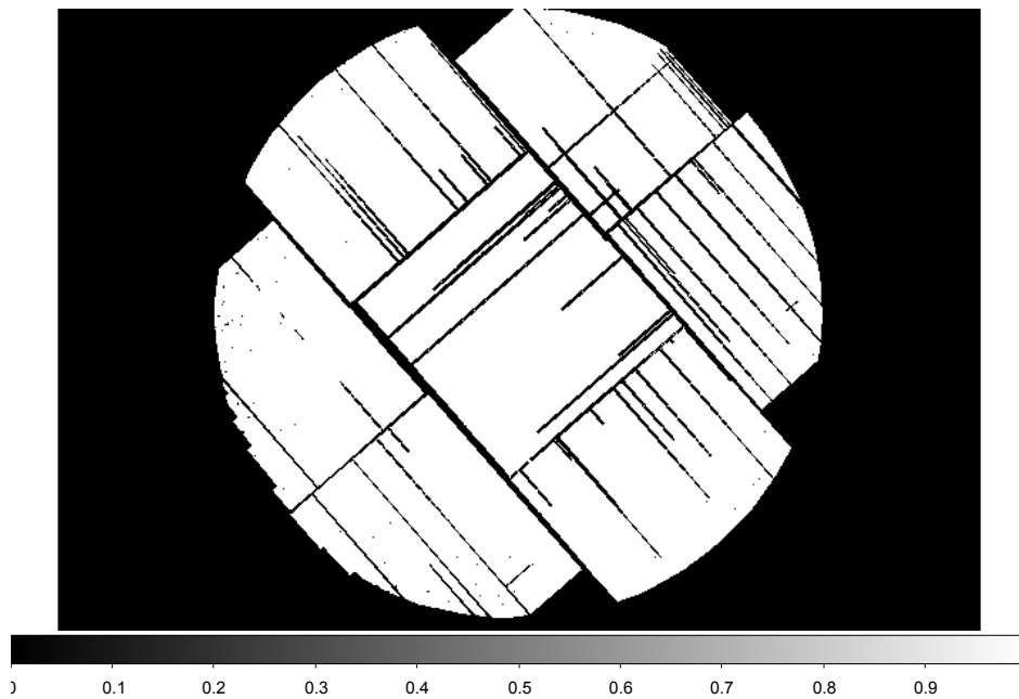
Figura 5.4. Máscara para la cámara EPIC MOS1, realizada a partir de el mapa de exposición de la observación del RSN G309.2-0.6 en el rango de energía 0.5 a 10 keV.
