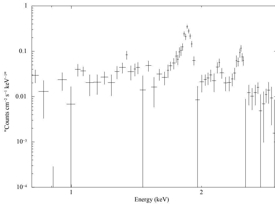
Figura 3.1. Espectro de origen térmico, correspondiente a la región central del RSN G309.2–0.6.
