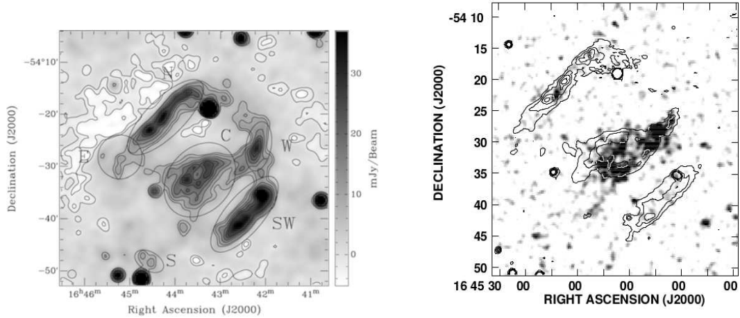
Figura 6.1. Izquierda: Mosaico del continuo de radio a 20cm (1384 MHz) del RSN G332.5–5.6 realizado con datos de ATCA, esta imagen fue tomada de Stupar et al. (2007). Derecha: Imagen de ROSAT PSPC en colores grises con contornos superpuestos correspondientes a la longitud de 20cm de la banda de radio, esta imagen fue tomada de Reynoso & Green (2007).
