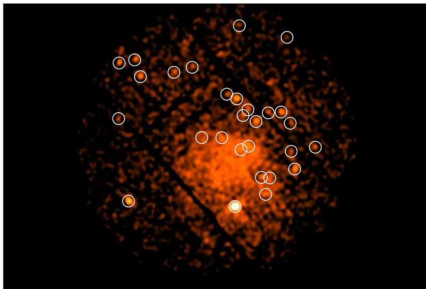
Figura 5.7. Fuentes detectadas en la cámara EPIC MOS1 para la observación de G309.2-0.6 en el rango de energía de 0.5 a 10 keV.
