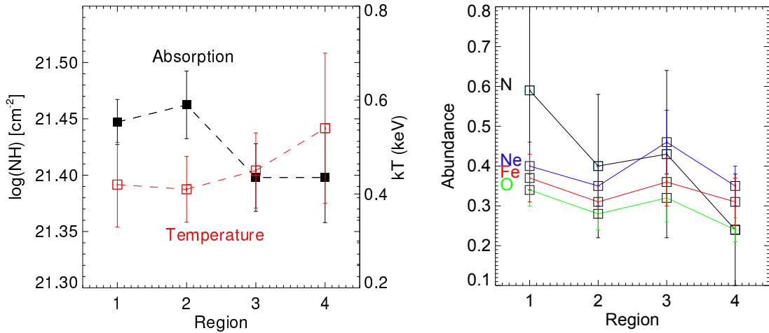
Figura 6.6. Parámetros de la emisión X, obtenidos del ajuste espectral, para cada una de las regiones. Izquierda: Los valores de absorción y temperatura tienen un comportamiento similar dentro de las barras de error, con un valor medio de \sim 2.6 \times 10^{21} \text{ cm}^{-2} y 0.45 keV, respectivamente. Derecha: las abundancias de N, Ne, Fe y O muestran valores sub-solares con un valor medio de \sim 0.4 \pm 0.07 .
