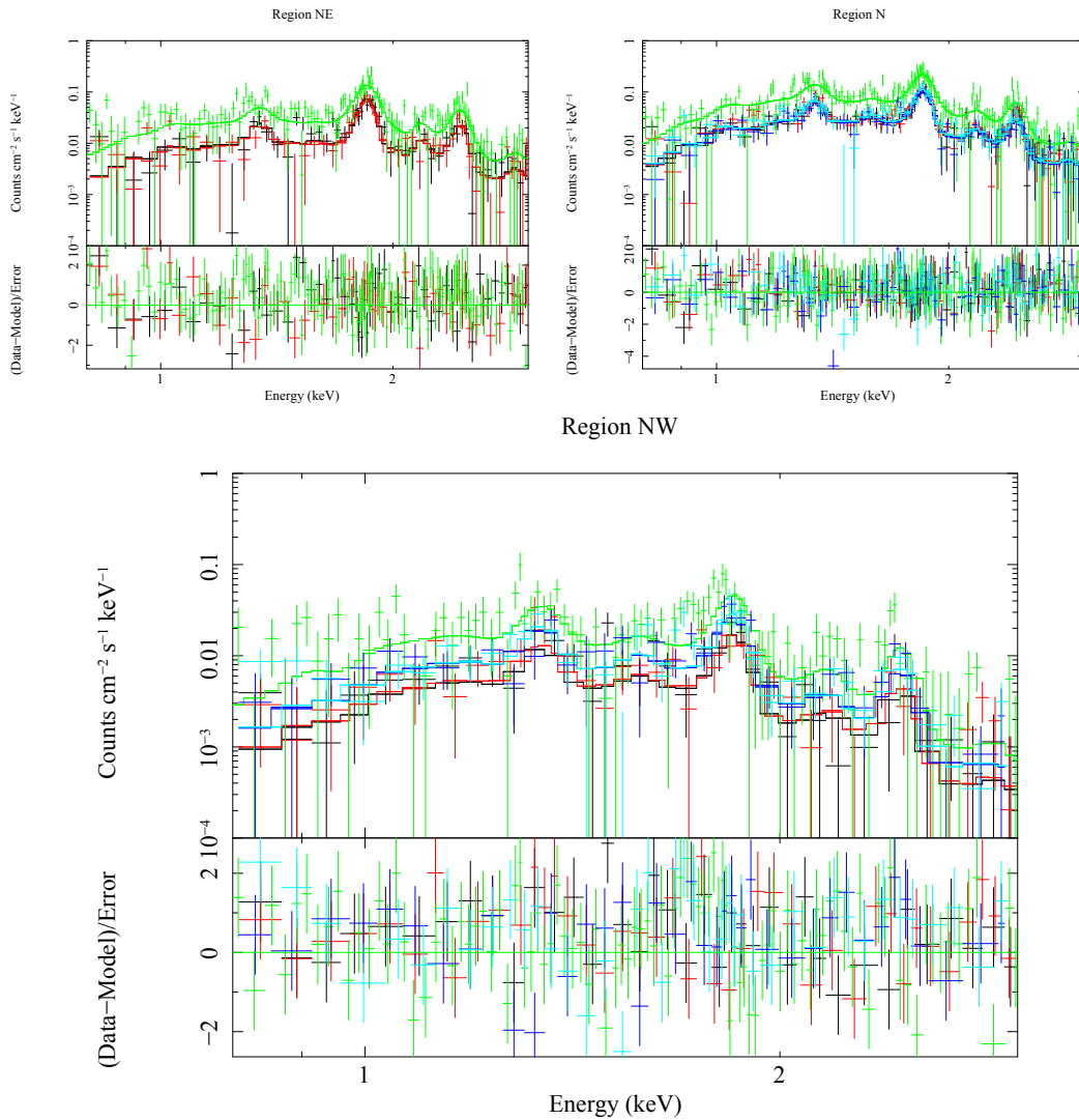
Figura 9.2. De izquierda a derecha: espectros de XMM-Newton correspondientes a las cámaras MOS1/2 y PN de las regiones NE, N y NW, respectivamente. Las líneas sólidas indican el modelo del mejor ajuste (ver Tabla 9.2). Los paneles inferiores representan los residuos del ajuste \chi^2 .
