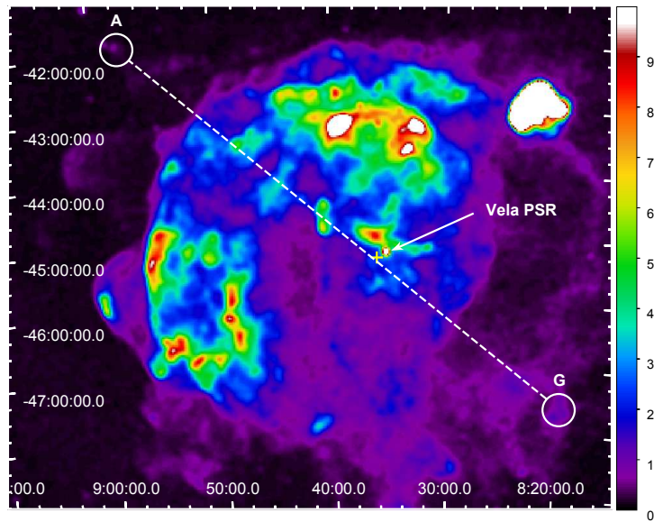
Figura 8.1. Imagen del RSN de Vela correspondiente a datos del relevamiento ROSAT All-Sky Survey en el rango de energía 0.44–2.04 keV. Los fragmentos A y G están indicados con círculos blancos y conectados con una línea punteada, la cual pasa cerca del púlsar de Vela y la posición de la explosión SN (marcada con una cruz amarilla). Esta última se calculó a partir de la edad y el movimiento propio del púlsar.
