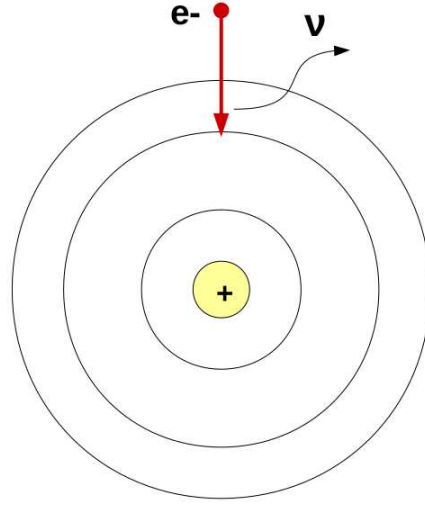
Figura 3.3. Esquema del proceso de recombinación radiativa. Un electrón con carga -e es capturado por un átomo, dándose lugar a una recombinación. Un fotón de frecuencia \nu es emitido, su energía es igual a la suma de la energía del electrón y la energía de ligadura del electrón recombinado.
