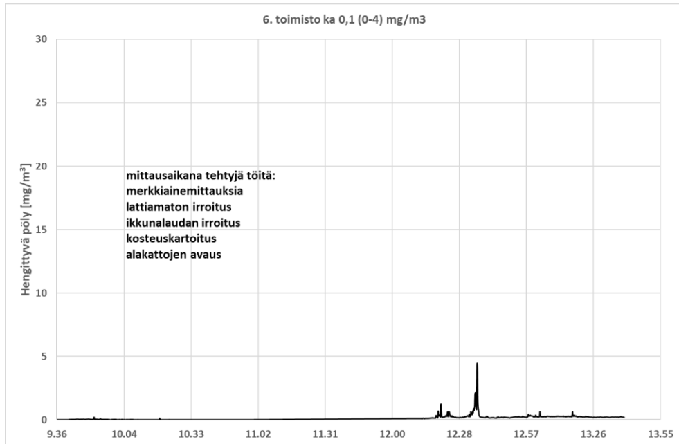
Kuva 10. Hengittävän pölyn pitoisuusvaihtelu asiantuntijan hengitysvyöhykkeellä kohteessa 6.
