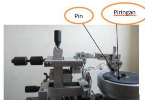
Gambar 2. Foto pengujian keausan
