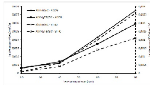
Gambar 6. Grafik laju keausan terhadap kecepatan putaran piringan Al 2 O 3 dan ST 40.
