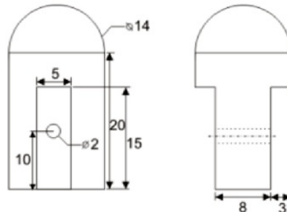
Gambar 1. Spesimen pin on disk
