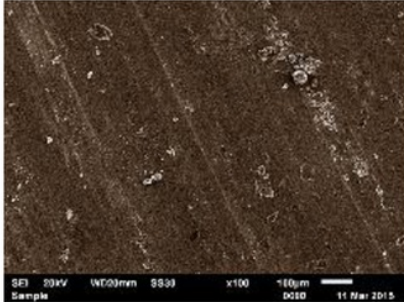
Gambar 8. Foto SEM AlSiMgTiB/SiC
