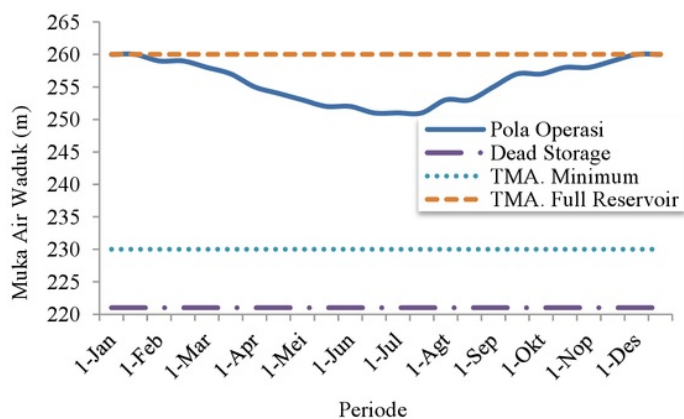
Gambar 14. Pola operasi Waduk Jatigede
