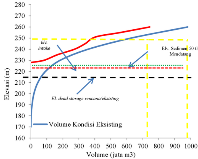
Gambar 15. Kurva tampungan waduk kondisi 50 tahun mendatang
