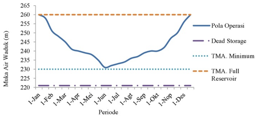
Gambar 17. Pola operasi Waduk Jatigede 50 tahun mendatang
