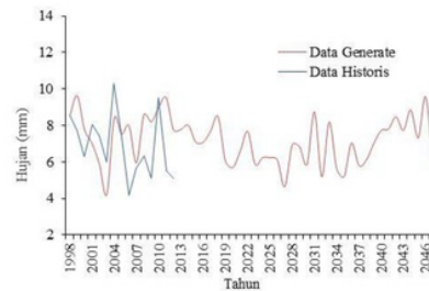
Gambar 9. Hasil generate data hujan Waduk Jatigede
