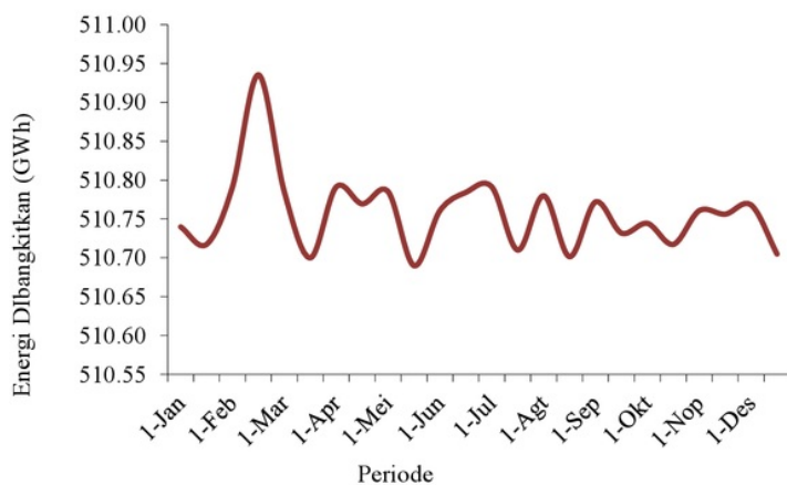
Gambar 13. Demand dan supply PLTA kondisi eksisting
