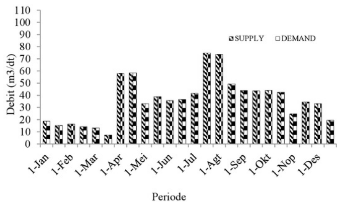
b) Gambar 12. (a) Demand dan supply air baku. b) Irigasi kondisi eksisting
