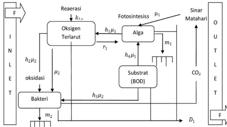
Gambar 1. Diagram Sistem Pengolahan Air Limbah Kolam Stabilisasi
