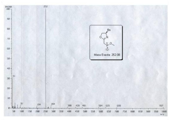
Figura 1. Espectro de MS ( \text{CI}^- ) de 14 .
