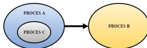
Obr. 2 Provázanost procesů [1]
