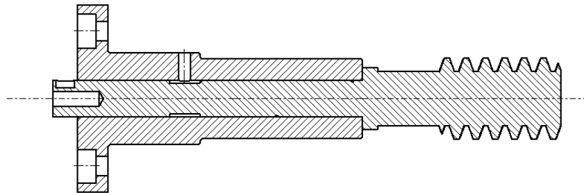
Obr. 24 Uložení šnekové hřídele v litinovém pouzdře
