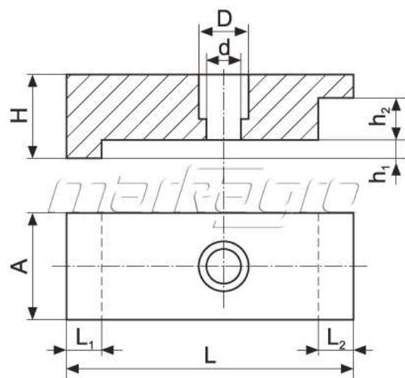
Obr. 11 Svěráková upínka FPZ 200 [10]
