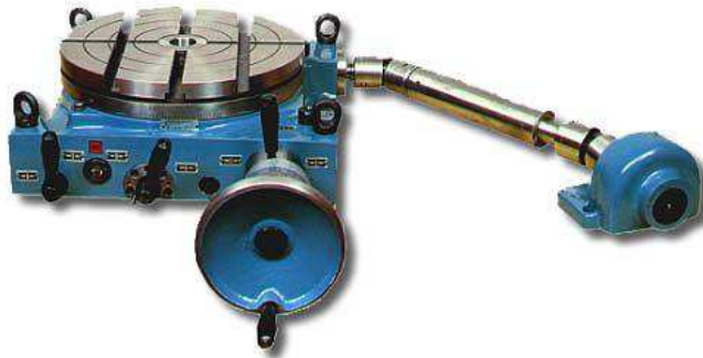
Obr. 1 – Otočný stůl TOS IMF 320 se strojím pohonem [1]
