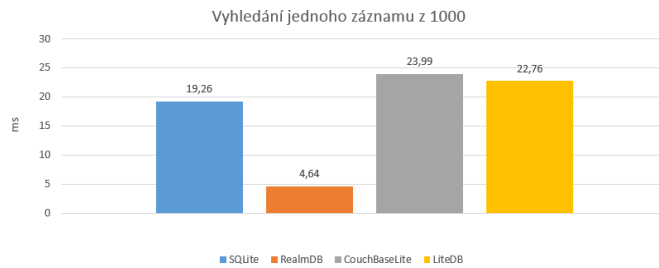
Obrázek 17: Graf pro načtení jednoho záznamu z 1000
