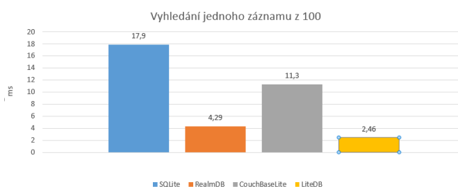
Obrázek 16: Graf pro načtení jednoho záznamu ze 100
