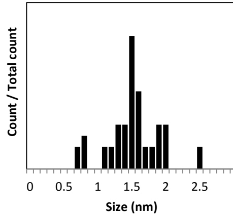
TiPt7.1%IE
