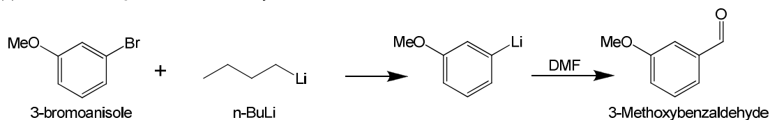
3-bromoanisole
