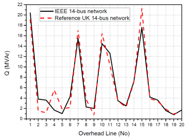
(d) reactive power flows comparison
