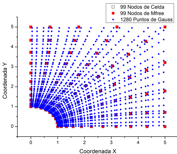
Figura 3: Malla.
