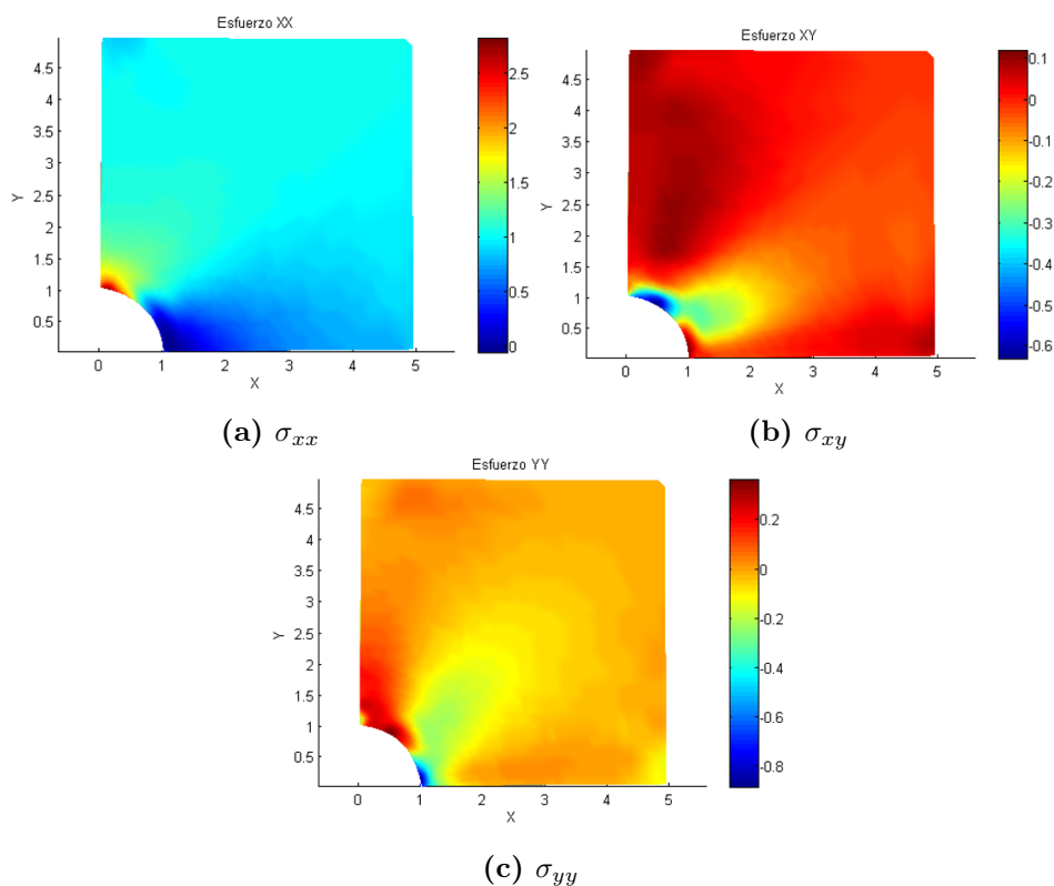
Figura 4: Solución numérica de los esfuerzos mediante RPIM (MQ), 99 nodos de campo.
