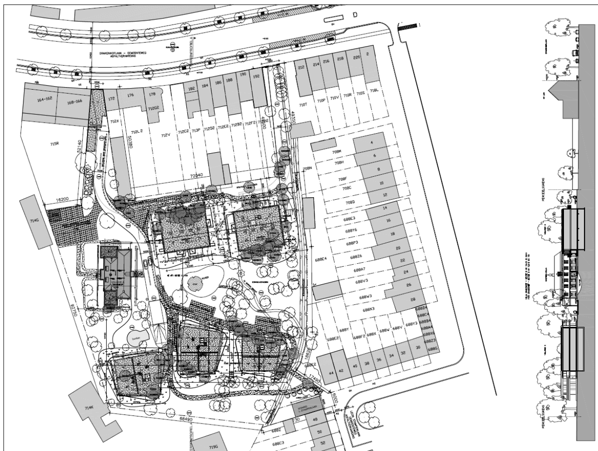
Fig. 6 Ontwerpplan van het onderzoeksgebied. (Crepain Binst Architecture)
