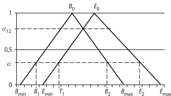
Рис. 2. Функції приналежності \mu_E , \mu_B ; фазова площина (E, B) для рівня \alpha
