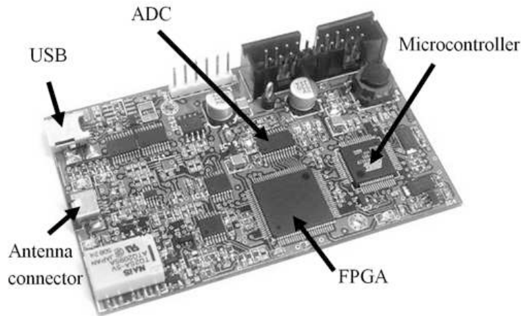
Fig. 2.1. The Proxmark III
