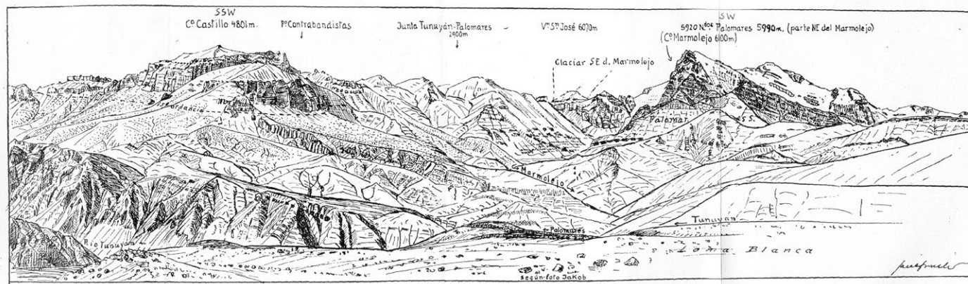
Figura 2: Panorama del río Palomares (vista al sur). El dibujo muestra la ubicación del Conglomerado Tunuyán en discordancia sobre rocas paleozoicas y cretácicas (Groeber 1951). Es un ejemplo de la calidad de las ilustraciones que acompañaron las publicaciones de Groeber.
