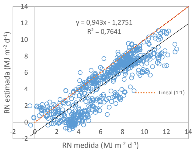
Figura 4. RN estimada con P-M con la corrección de R_{so} por la transmisividad frente a RN medida (con y sin enalado años 1996 a 2001).
