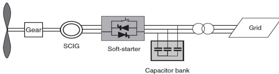
FIGURA 5 GENERADOR DE INDUCCIÓN CON ROTOR DE JAULA DE ARDILLA ACCIONADO POR UN ROTOR EÓLICO DE VELOCIDAD CONSTANTE.
