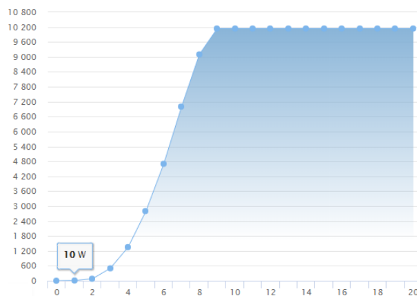
FIGURA 19 CURVA DE POTENCIA CONTRA VELOCIDAD.
