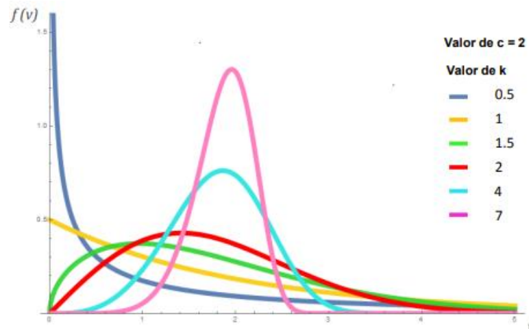
FIGURA 10 GRAFICA DE LA FUNCIÓN DE PROBABILIDAD DE WEIBULL.
