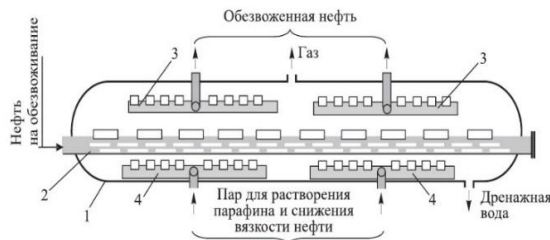
Рис. 1 Горизонтальный отстойник конструкции «ВНИИнефтемаш» и «Гипротюменнефтегаз»: 1 — корпус; 2 — коллектор ввода нефти на обезвоживание; 3 — коллектор вывода обезвоженной нефти; 4 — коллектор подачи пара для растворения парафина [3].
