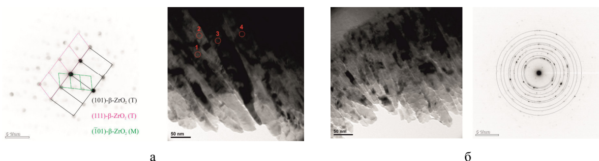
Рис. 1. Электронно-микроскопическое изображение многослойных покрытий на основе Zr-Y-O в исходном состоянии (а); при отжиге 900^\circ\text{C} в течение 20 минут (б): светлопольные изображения поперечного сечения; микродифракционные картины и схемы ее индицирования
