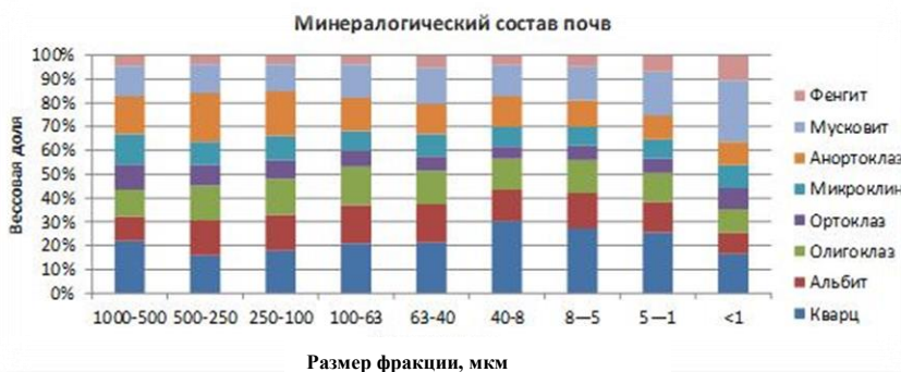
Рис. 2 Распределение минералов по гранулометрическим фракциям почв водотока шт. 176
