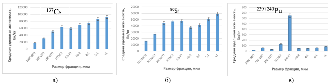
Рис. 1 Распределение радионуклидов по гранулометрическим фракциям почв водотока шт. 176
