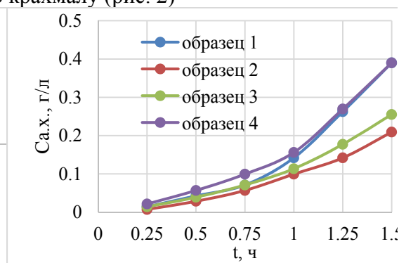
Рис.2. Зависимость концентрации активного хлора от времени в разбавленном растворе гидролизата рисовой шелухи
