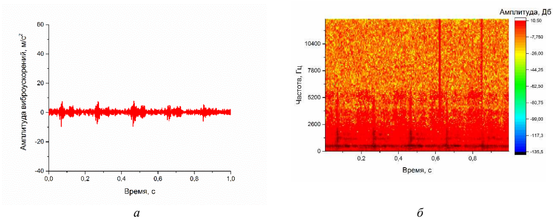
Рис. 3. Изменение амплитуды виброускорений (а) и STFT картина распределения частот колебаний (б) во времени при трении неупрочненного материала
