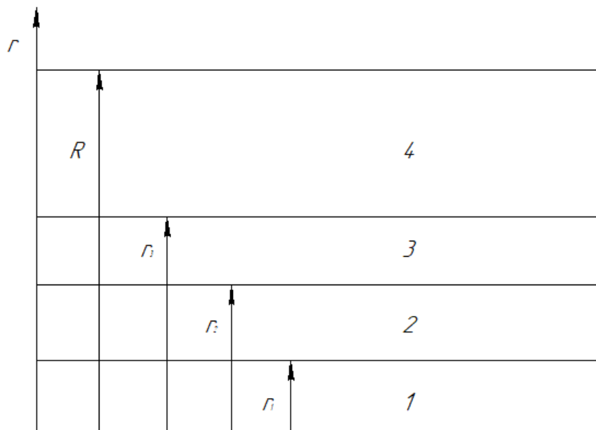
Рисунок 17 – Область решения задачи. 1 – корень, 2 – слой почвы, 3 – слой ЛГМ, 4 – слой воздуха
