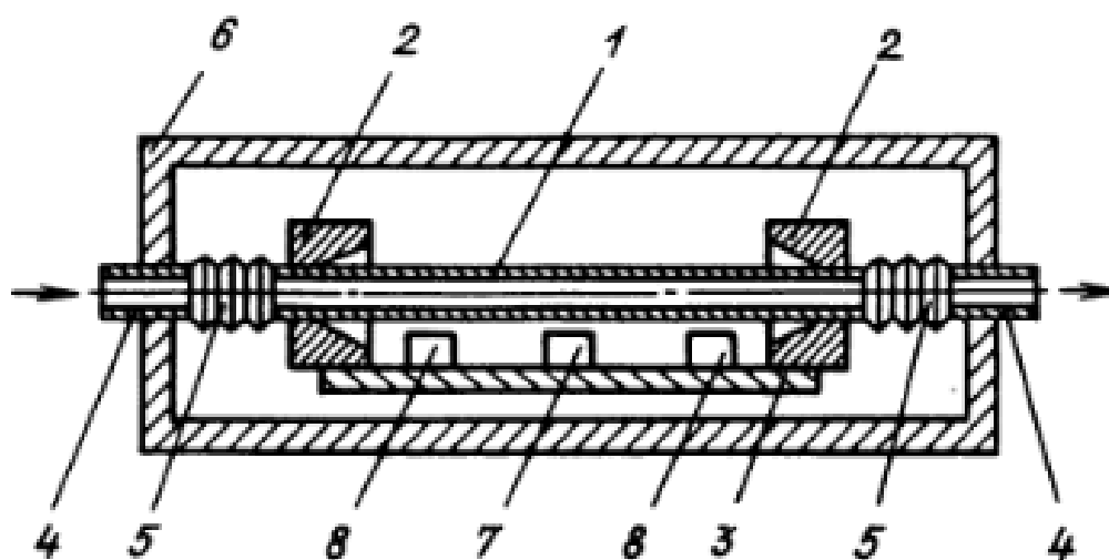
Рисунок 1 – однотрубчатый вибрационный плотномер.
