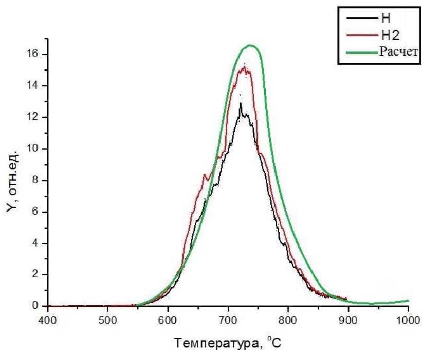
Рисунок 22 Моделирование термостимулированного выхода водорода, ТСГВ_Ti_Bт1-0
