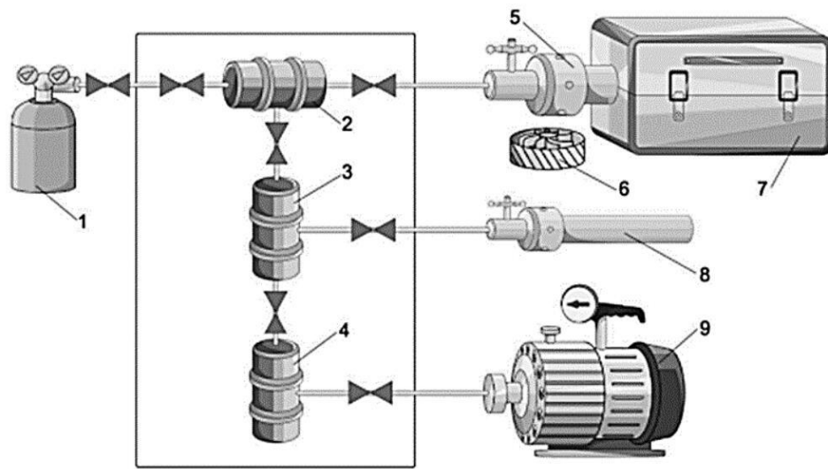
Рисунок 2 Схема установки для насыщения металлических образцов из метода Сиверты. 1 – баллон с водородом; 2, 3, 4 – каналы подачи/откачки водорода; 5 – большая камера (175 см 3 ); 6 – вентилятор; 7 – печь; 8 – малая камера; 9 – вакуумный насос
