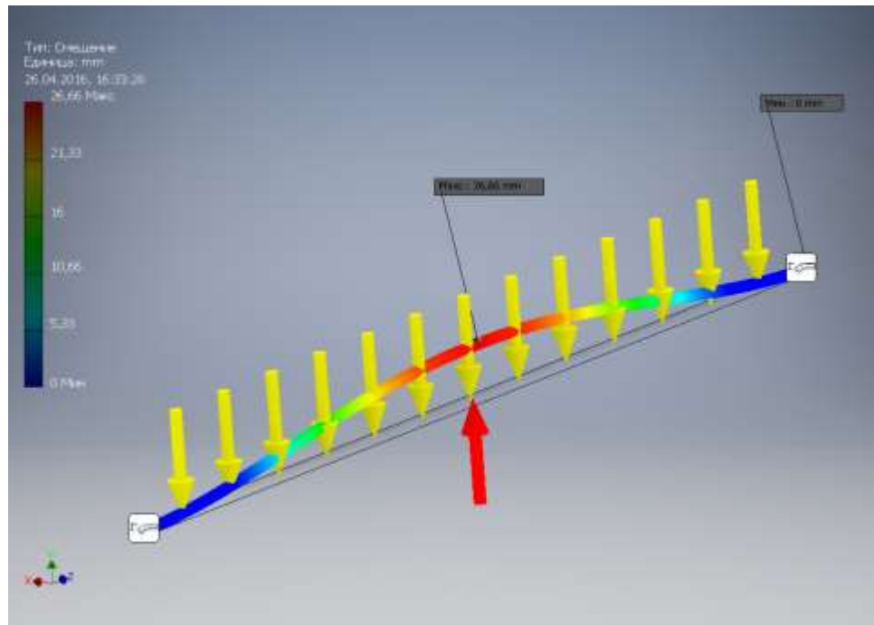
Рисунок 3.12 – Смещение
