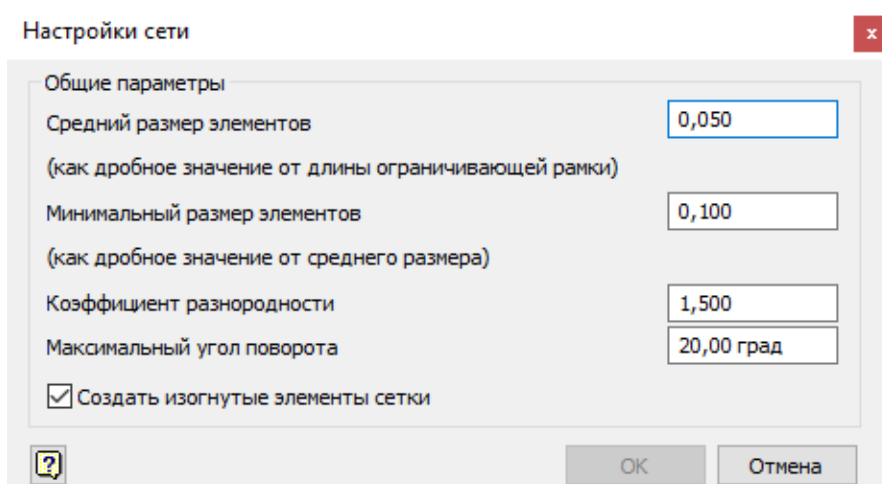
Рисунок 3.24 – Настройка сетки
