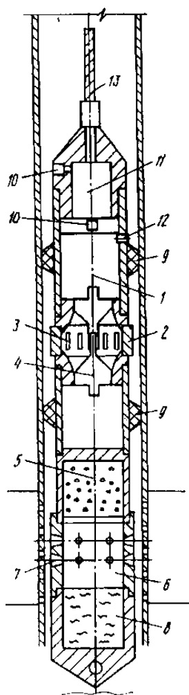
Рисунок 12 - Устройство для ГРП
