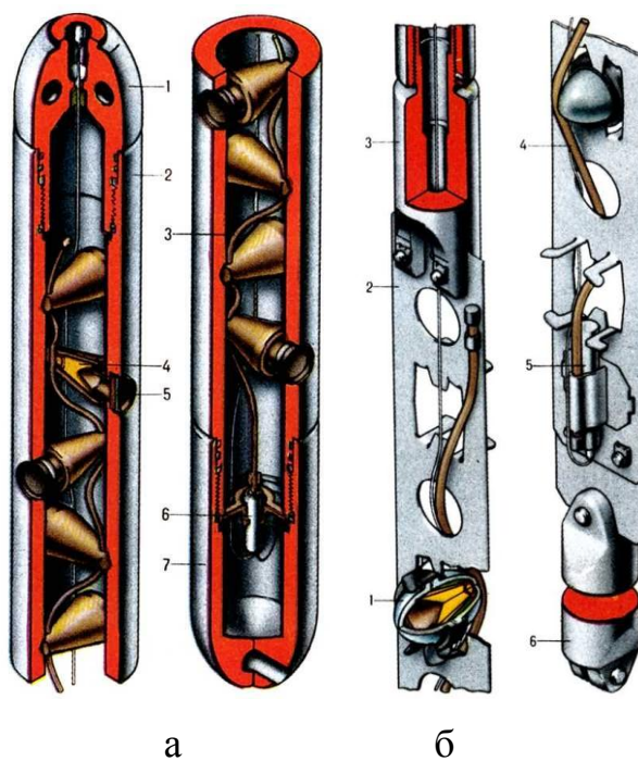
Рисунок 14 - Кумулятивные перфораторы. а - корпусный перфоратор: 1 - головка; 2 - корпус; 3 - детонирующий шнур; 4 - кумулятивный заряд; 5 - герметизирующее уплотнение; б - взрывной патрон; 7 – наконечник; б – бескорпусный перфоратор: 1 - кумулятивный заряд в стеклянной и ситалловой оболочках; 2 - лента; 3 - головка; 4 - детонирующий шнур; 5 - взрывной патрон; 6 - груз.
