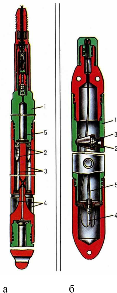
Рисунок 15 - Пулевые перфораторы. а – перфоратор с горизонтальным стволом: 1 - корпус; 2 - пробка; 3 - заряд; 4 - патрон предохранительного действия; 5 - детонирующий шнур; б – перфоратор с вертикальным стволом: 1 - корпус; 2 - пуля; 3 - канал перфоратора; 4 - отклоняющий участок; 5 - пороховой заряд
