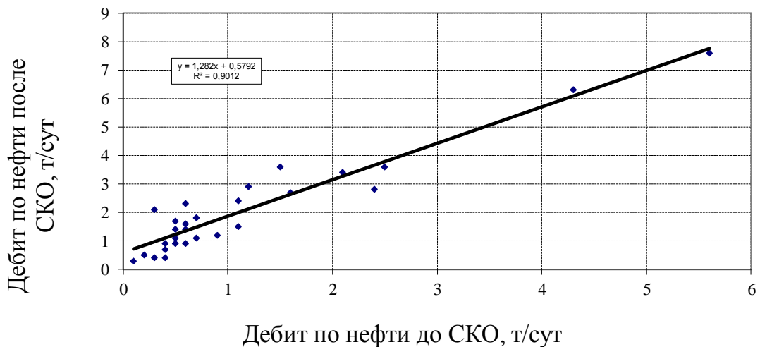
Рисунок 9 – Зависимости дебита нефти после проведения СКО от дебита нефти до проведения СКО
