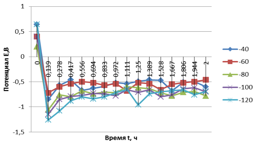
Рис. 1. Разрядные E,t- кривые электрода, изготовленного из Ni(OH)_2 полученного при добавке C_{пк}=50 г/л при i=40-120 мА/см 2
