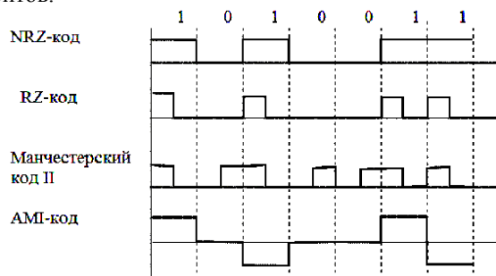
Рис. 1. Самосинхронизирующиеся коды
