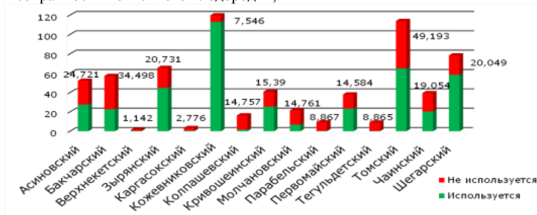
Рис. 1. Площади используемых и залежных земель по районам Томской области в 2016 г., тыс. га.
