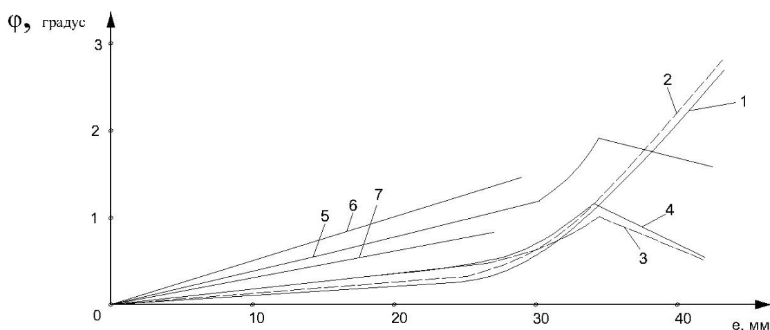
Рис. 1. Экспериментальные кривые зависимости угла перекоса забоя от эксцентриситета приложения удара: кривая I – порода мрамор, масса ударника m_y=6,5 кг, высота ударника H_y=12 см, высота сбрасывания ударника h_c=2,9 м; II – порода мрамор, h_c=2 м, остальные параметры аналогичны кривой I; III – порода мрамор, m_y=3,5 кг, H_y=7 см, h_c=2,9 м; IV – материал дюралюминий, параметры ударной системы те же; V, VII – порода гранит, параметры ударной системы те же; VI – порода мрамор, параметры ударной системы те же.
