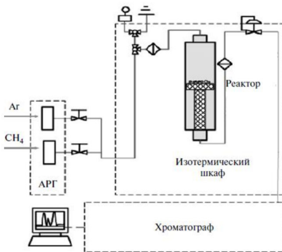
Рис. 1. Принципиальная схема лабораторной установки
