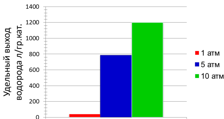
Рис. 2. Удельный выход водорода при различных давлениях
