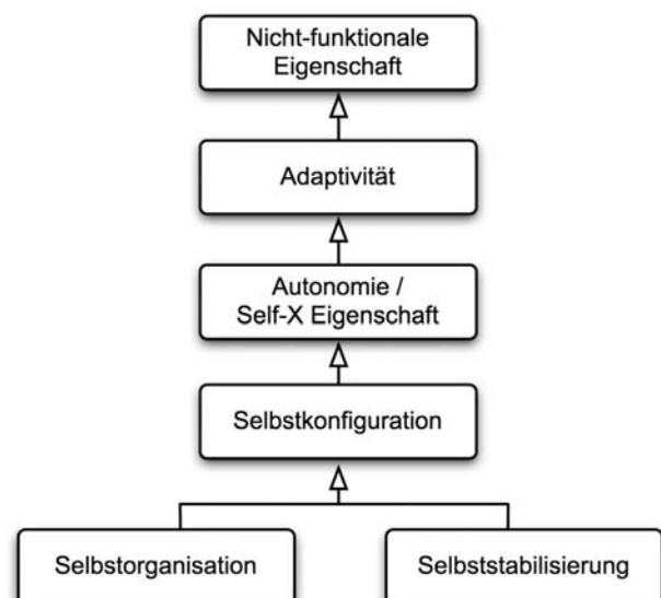
Abb. 3. Konzeptionelles Modell von Adaptivität und Autonomie.
