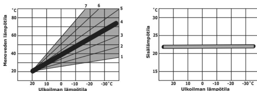
Kuva 8. Säätokäyrä on asetettu oikein, kun huonelämpötila pysyy tasaisena (1, s. 10).
