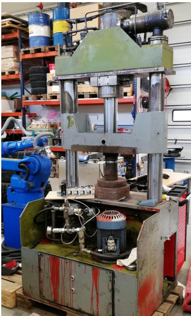
KUVA 1. Hydrauliprässin runko alkuperäisillä osilla
