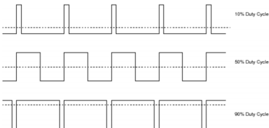
KUVA 17. Erilaisia PWM-signaaleja
