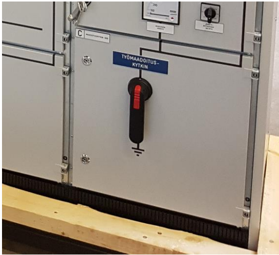
KUVA 9. Kennokeskuksen työmaadoituskytkin
