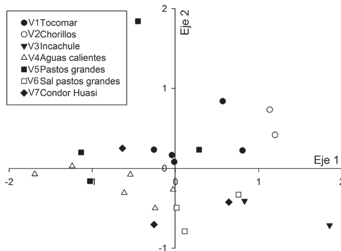
Fig. 2. Diagrama de ordenamiento de los sitios de muestreo de las diferentes vegas a lo largo de dos ejes del NMDS. Fig. 2. Ordination of the sampling sites of each peatbogs along NMDS axes.
