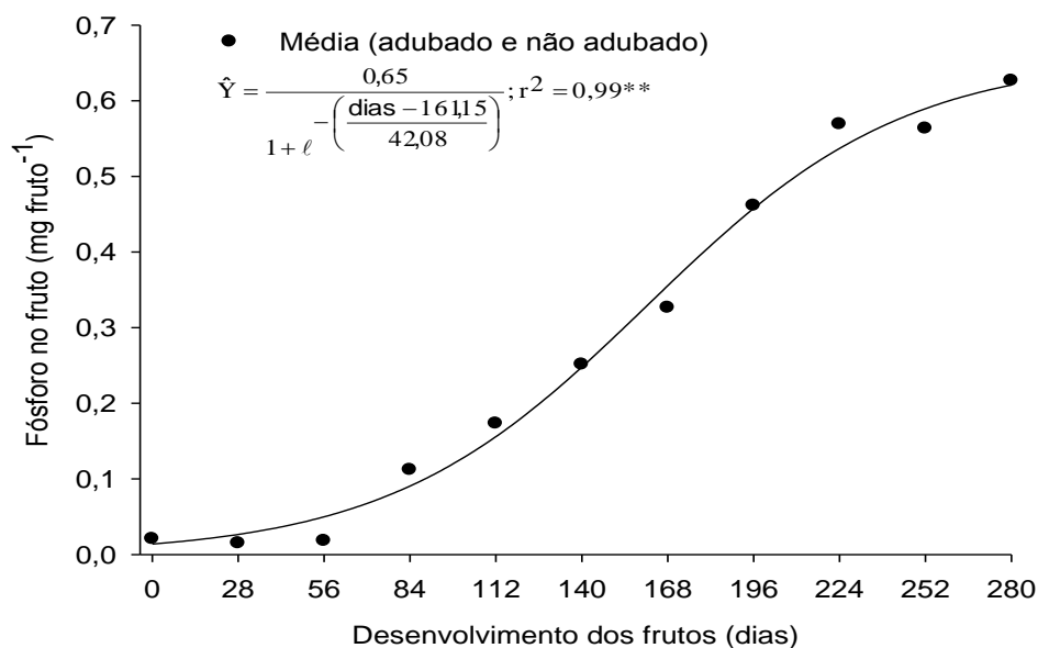
FIGURA 4. Acúmulo de fósforo em frutos de cafeeiro coletados desde a fase chumbinho até a maturação. As barras representam o erro padrão da média.
