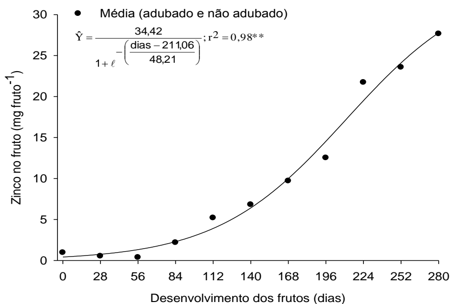
FIGURA 7. Acúmulo de zinco em frutos de café conilon coletados desde a fase chumbinho até a maturação. As barras representam o erro padrão.
