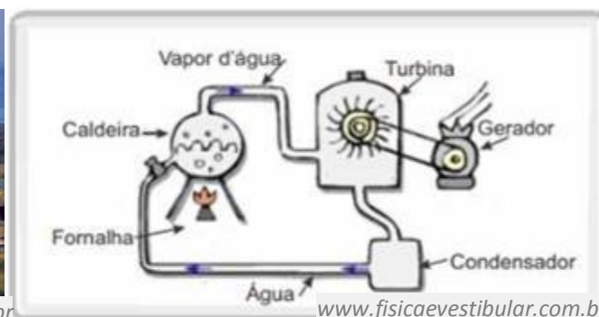
Figura 27. Na foto de termoelétrica, repare na geração de fumaça e na proximidade de mar, para uso de água abundante para resfriamento da condensadora, como no esquema ao lado; esquema de funcionamento (repare que a diferença entre esta usina e a hidroelétrica, é o que faz girar o gerador).
