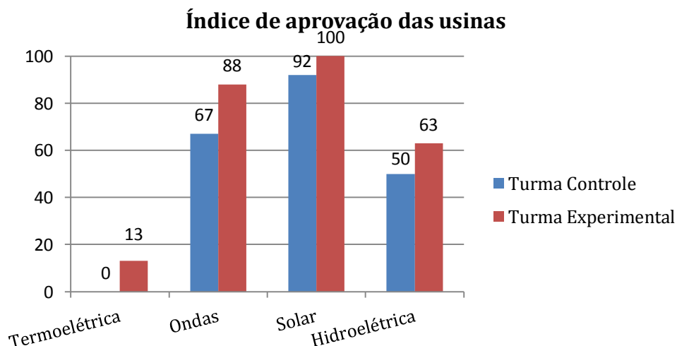
Figura 4.19: Gráfico dos níveis de aprovação dos alunos por usina.
