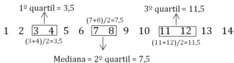
Figura 3.33: Exemplo de cálculo dos quartis.
