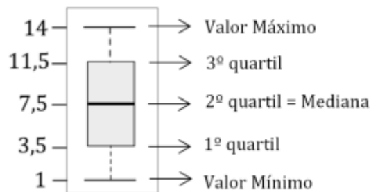
Figura 3.34: Os quartis num exemplo de boxplot.
