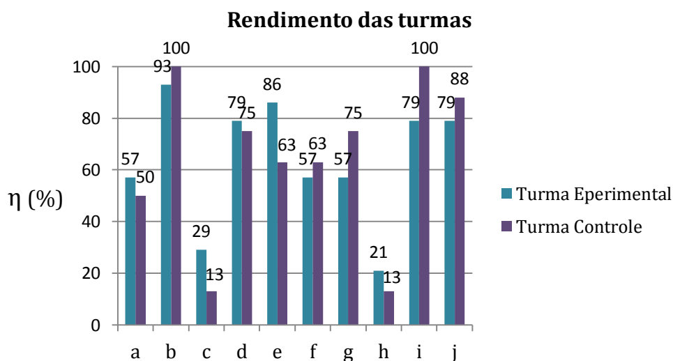
Figura 4.17: Gráfico do rendimento das turmas por item da Questão 9 do Pós Teste.
