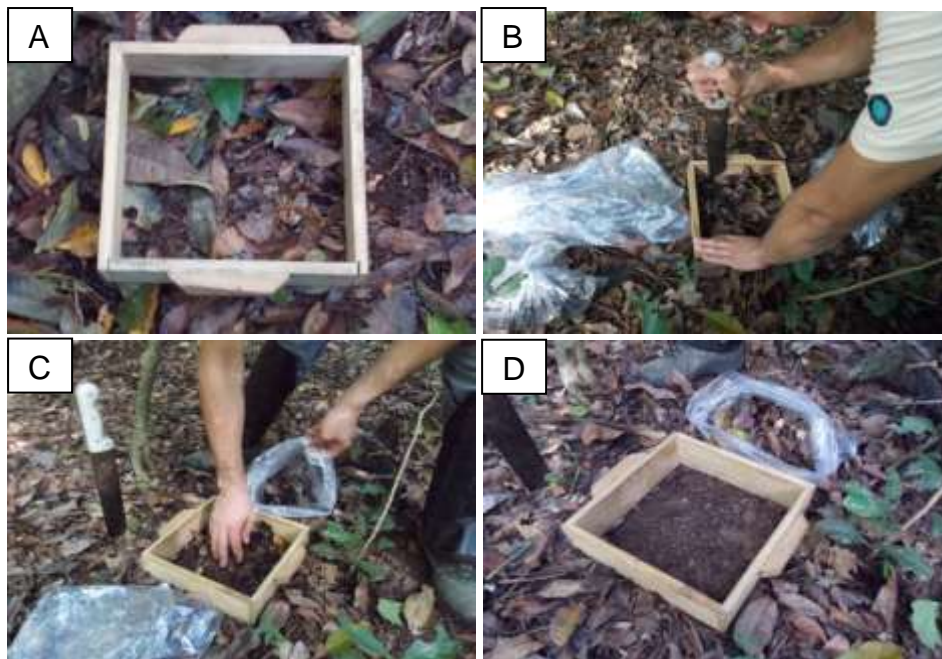
Figura 2. 2 - (A) Gabarito para coleta de serapilheira acumulada e (B, C, D) coleta da serapilheira acumulada.
