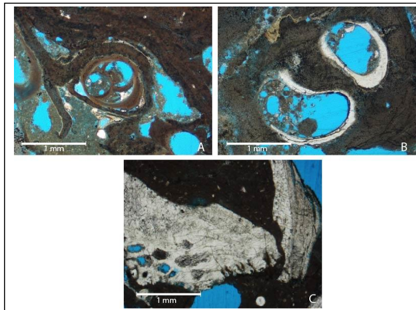
Figura 10: Organismos com funções secundárias no crescimento do recife também encontrados nas lâminas petrográficas, como (A) Foraminíferos, (B) Vermetídeos e (C) Moluscos (bivalves e gastrópodes).
