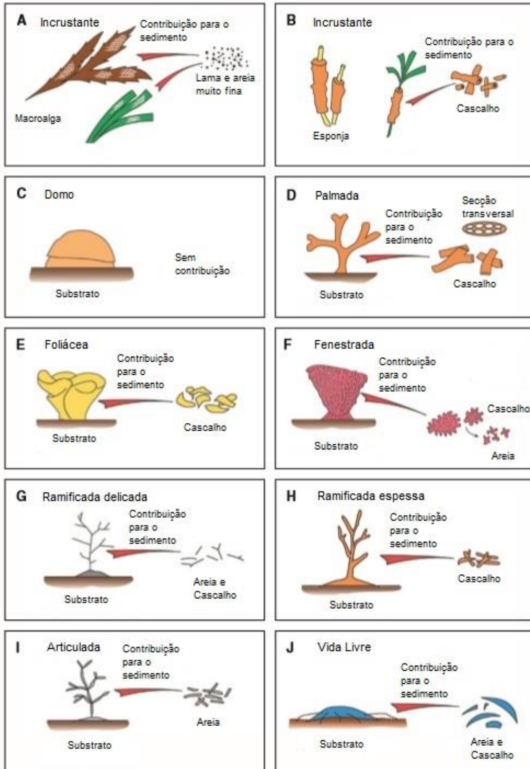
Figura 11: Típicas formas coloniais de briozoários e suas contribuições para o sedimento. Formas (A) e (B) incrustantes, (C) em formato de domo, (D) palmada, (E) foliácea, (F) fenestrada, (G) ramificada delicada, (H) ramificada espessa, (I) articulada e (J) de vida livre. Fonte: Modificada de Taylor e James (2013).
