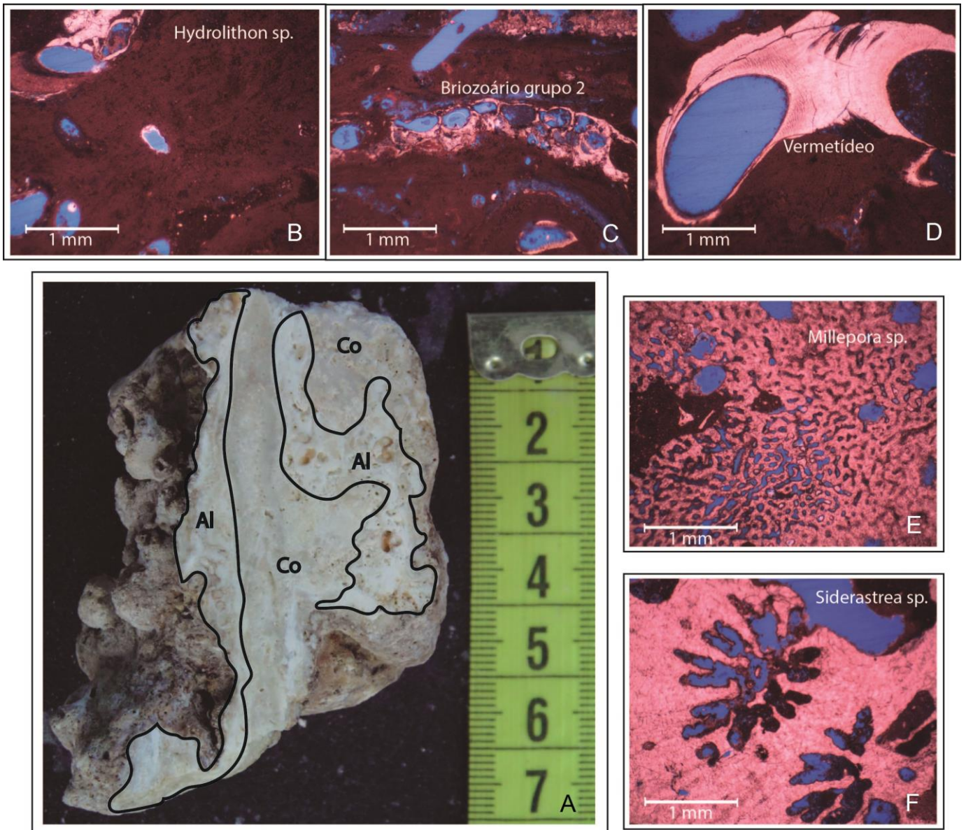
Figura VI: Fragmento 6P, localizado próximo ao centro do testemunho vertical LG-AB-DR 06, e suas respectivas imagens de lâminas petrográficas. (A) Imagem macroscópica do fragmento recifal, onde são evidenciados Alga Calcária (Al) e Coral (Co). (B) Imagem de lâmina microscópica evidenciando alga calcária da espécie Hydrolithon sp. (C) Imagem de lâmina microscópica evidenciando Briozoário grupo 2. (D) Imagem de lâmina microscópica evidenciando vermetídeo. (E) Imagem de lâmina microscópica evidenciando coral da espécie Millepora sp. e (F) Imagem de lâmina microscópica evidenciando coral da espécie Siderastrea sp.
