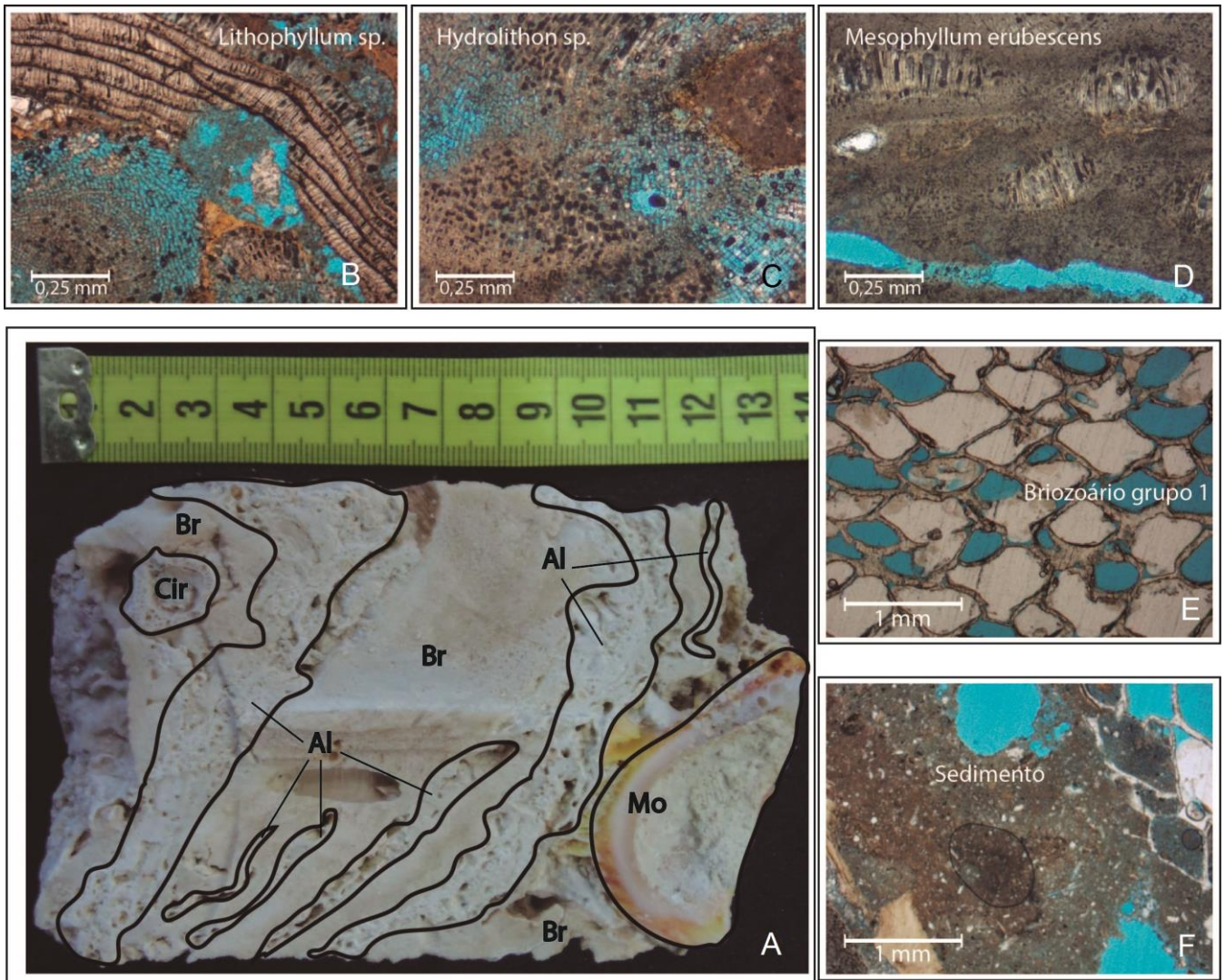
Figura VII: Fragmento 3A, localizado no topo do testemunho horizontal LG-AB-DR 03, e suas respectivas imagens de lâminas petrográficas. (A) Imagem macroscópica do fragmento recifal, onde são evidenciados Alga Calcária (Al), Briozoário (Br), Molusco (Mo) e Cirrípede (Cir). (B) Imagem de lâmina microscópica evidenciando alga calcária da espécie Lithophyllum sp. (C) Imagem de lâmina microscópica evidenciando alga calcária da espécie Hydrolithon sp. (D) Imagem de lâmina microscópica evidenciando alga calcária da espécie Mesophyllum erubescens . (E) Imagem de lâmina microscópica evidenciando Briozoário grupo 1. e (F) Imagem de lâmina microscópica evidenciando sedimento fino.
