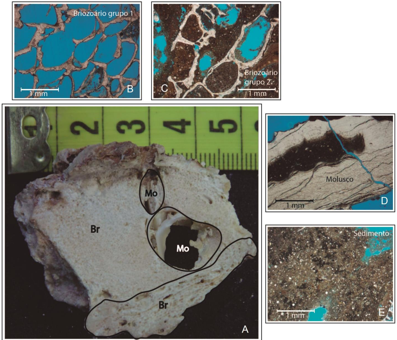
Figura IX: Fragmento 7C, localizado próximo ao topo do testemunho horizontal LG-AB-DR 07, e suas respectivas imagens de lâminas petrográficas. (A) Imagem macroscópica do fragmento recifal, onde são evidenciados Briozoário (Br) e Molusco (Mo). (B) Imagem de lâmina microscópica evidenciando Briozoário grupo 1. (C) Imagem de lâmina microscópica evidenciando Briozoário grupo 2. (D) Imagem de lâmina microscópica evidenciando Molusco. e (E) Imagem de lâmina microscópica evidenciando sedimento fino.
