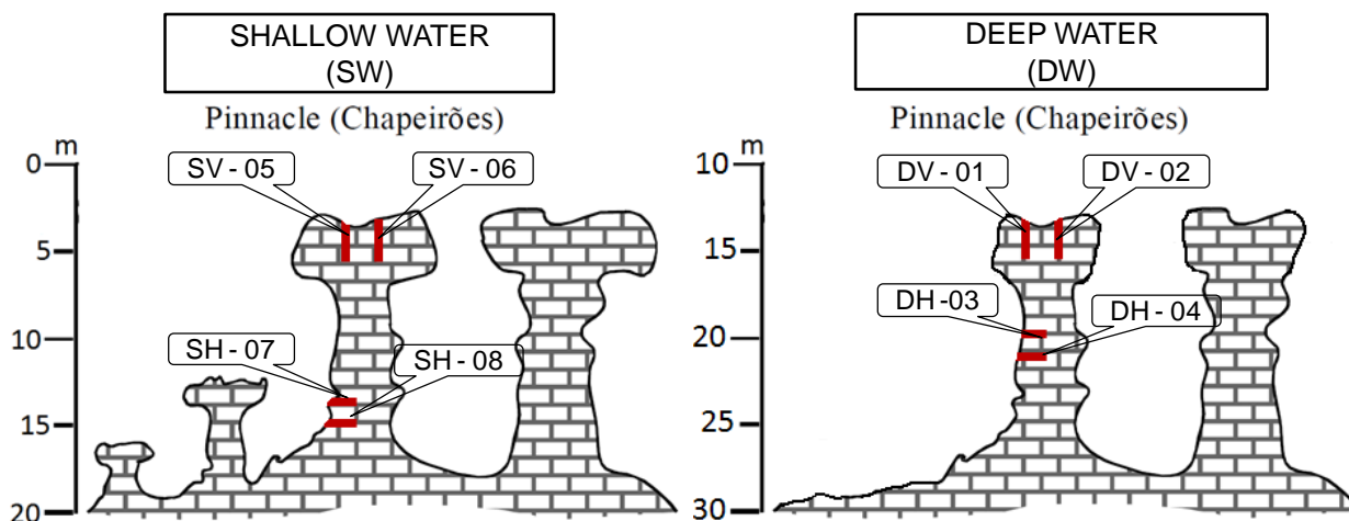
Figura 3: Imagem ilustrando as perfurações nos dois ambientes recifais identificados como “Deep Water” e “Shallow Water”. Em vermelho são identificados os testemunhos SV-05, SV-06, SH-07 e SH-08 no ambiente “Shallow Water” e DV-01, DV-02, DH-03 e DH-04 no ambiente “DW”. FONTE: Modificado de LEÃO et al., 2003.
