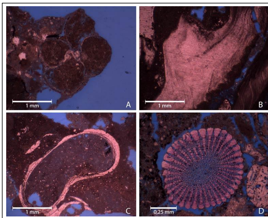
Figura 7: Organismos com funções secundárias no crescimento do recife também encontrados nas lâminas petrográficas, como (A) Foraminíferos, (B) Moluscos como bivalves e gastrópodes, (C) Vermetídeos e (D) Fragmentos de Equinodermas.
