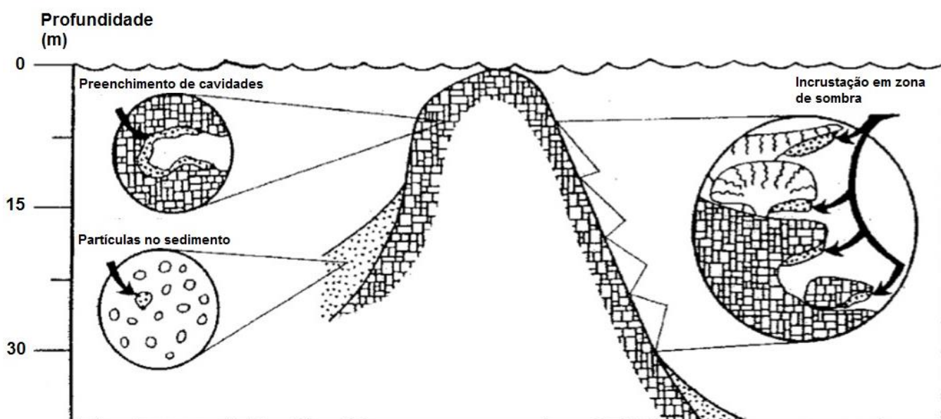
Figura 12: Ilustração da presença dos briozoários nas regiões abrigadas dos recifes modernos. Fonte: Modificada de Cuffey (1977).
