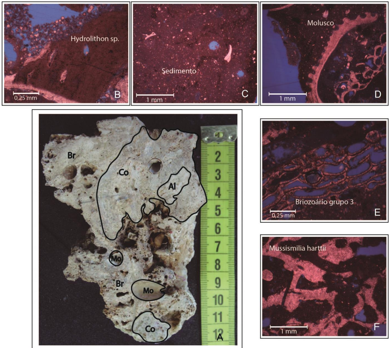
Figura II: Fragmento 2C, localizado próximo ao topo do testemunho vertical LG-AB-DR 02, e suas respectivas imagens de lâminas petrográficas. (A) Imagem macroscópica do fragmento recifal, onde são evidenciados Briozário (Br), Alga Calcária (Al), Coral (Co), e Molusco (Mo). (B) Imagem de lâmina microscópica evidenciando alga calcária da espécie Hydrolithon sp. (C) Imagem de lâmina microscópica evidenciando sedimento fino. (D) Imagem de lâmina microscópica evidenciando Molusco, (E) Imagem de lâmina microscópica evidenciando Briozário grupo 3 e (F) Imagem de lâmina microscópica evidenciando coral da espécie Mussismilia harttii .
