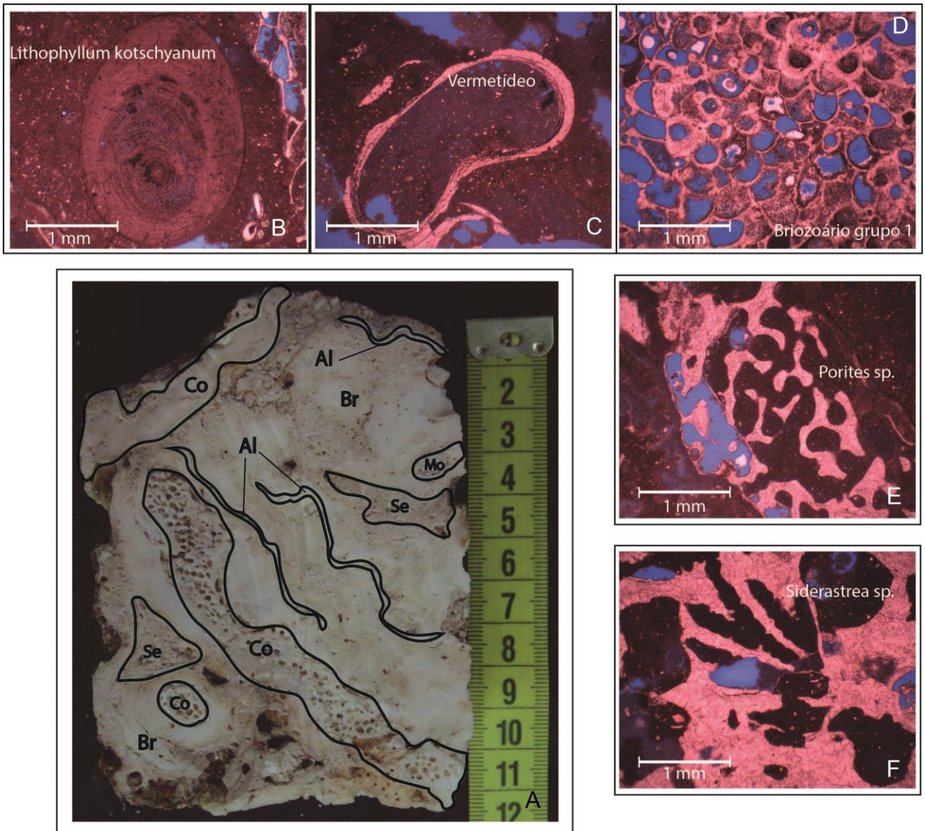
Figura III: Fragmento 5B, localizado próximo ao topo do testemunho vertical LG-AB-DR 05, e suas respectivas imagens de lâminas petrográficas. (A) Imagem macroscópica do fragmento recifal, onde são evidenciados Briozoário (Br), Alga Calcária (Al), Coral (Co), Sedimento fino (Se) e Molusco (Mo). (B) Imagem de lâmina microscópica evidenciando alga calcária da espécie Lithophyllum kotschyannum . (C) Imagem de lâmina microscópica evidenciando vermetídeo. (D) Imagem de lâmina microscópica evidenciando Briozoário grupo 1, (E) Imagem de lâmina microscópica evidenciando coral da espécie Porites sp. e (F) Imagem de lâmina microscópica evidenciando coral da espécie Siderastrea sp.
