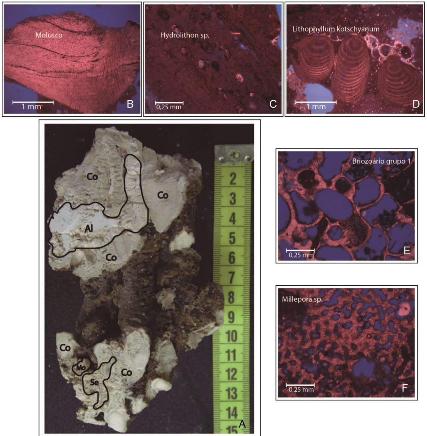
Figura IV: Fragmento 5H, localizado próximo ao centro do testemunho vertical LG-AB-DR 05, e suas respectivas imagens de lâminas petrográficas. (A) Imagem macroscópica do fragmento recifal, onde são evidenciados Alga Calcária (Al), Coral (Co), Sedimento fino (Se) e Molusco (Mo). (B) Imagem de lâmina microscópica evidenciando Molusco. (C) Imagem de lâmina microscópica evidenciando alga calcária da espécie Hydrolithon sp. (D) Imagem de lâmina microscópica evidenciando alga calcária da espécie Lithophyllum kotschyanum . (E) Imagem de lâmina microscópica evidenciando Briozoário grupo 1 e (F) Imagem de lâmina microscópica evidenciando coral da espécie Millepora sp.
