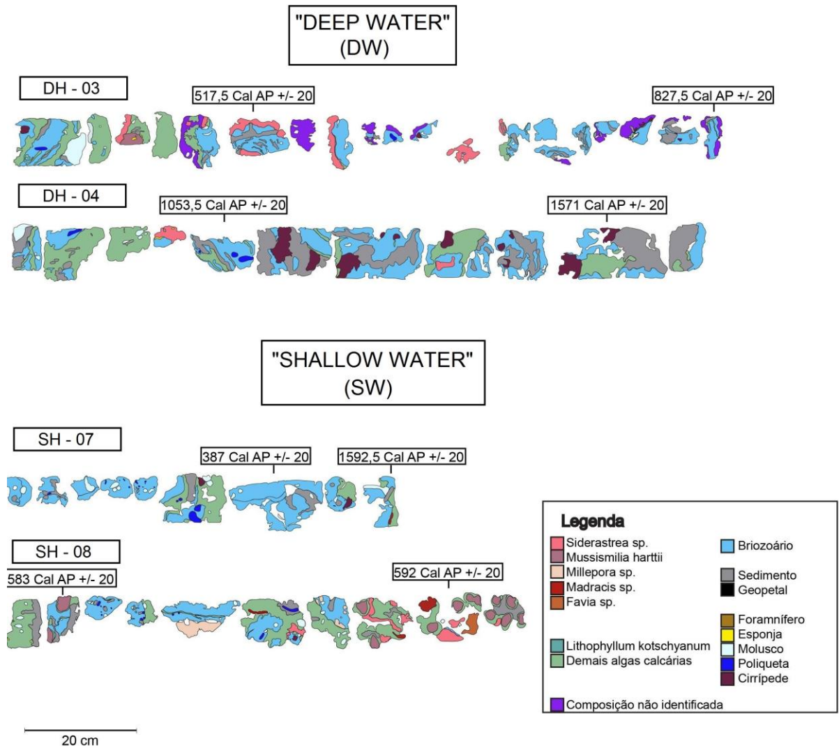
Figura 8: Assemblage dos organismos encontrados nos testemunhos horizontais dos ambientes Shallow Water (SW) e Deep Water (DW). Testemunhos recifais DH - 03, DH - 04, SH - 07 e SH - 08. Em quadros pretos são apresentadas idades calibradas em 2\sigma expressas em "Cal AP" +/- 20, ou seja, idades calendário antes do presente com erro de até 20 anos.
