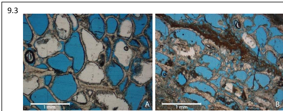
Figura 9: Espécies de corais, algas e briozoários encontradas nos testemunhos horizontais dos ambientes Shallow Water (SW) e Deep Water (DW). Em 9.1 são apresentados os corais (A) e (B) Siderastrea sp. , (C) hidrocoral Millepora sp. , (D) Mussismilia harttii . Em 9.2 são apresentadas as algas (A) Hydrolithon sp. , (B) e (C) Lithophyllum sp. , (D) Lithophyllum kotschyanum , (E) Mesophyllum erubescens . e (F) Sporolithon episporum . Já em 9.3 são apresentados os briozoários (A) Briozoário Grupo 1 e (B) Briozoário Grupo 2.
