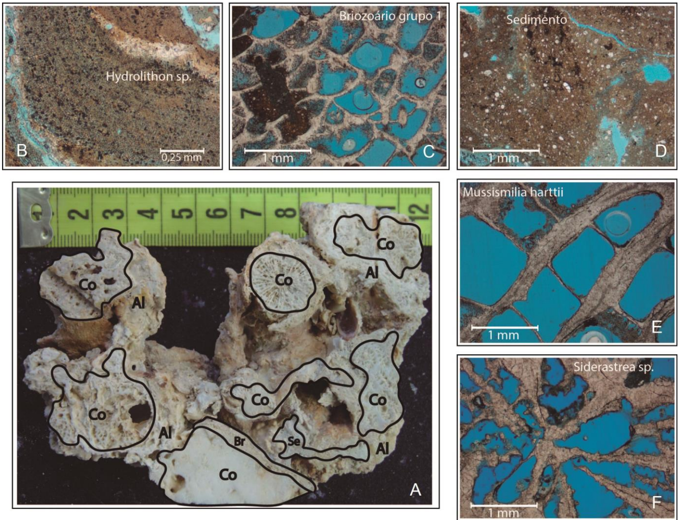
Figura XI: Fragmento 8I, localizado próximo à base do testemunho horizontal LG-AB-DR 08, e suas respectivas imagens de lâminas petrográficas. (A) Imagem macroscópica do fragmento recifal, onde são evidenciados Briozoário (Br), Coral (Co), Alga calcária (Al) e Sedimento fino (Se). (B) Imagem de lâmina microscópica evidenciando alga calcária da espécie Hydrolithon sp. (C) Imagem de lâmina microscópica evidenciando Briozoário grupo 1. (D) Imagem de lâmina microscópica evidenciando sedimento fino. (E) Imagem de lâmina microscópica evidenciando coral da espécie Mussismilia harttii . e (F) Imagem de lâmina microscópica evidenciando coral da espécie Siderastrea sp.
