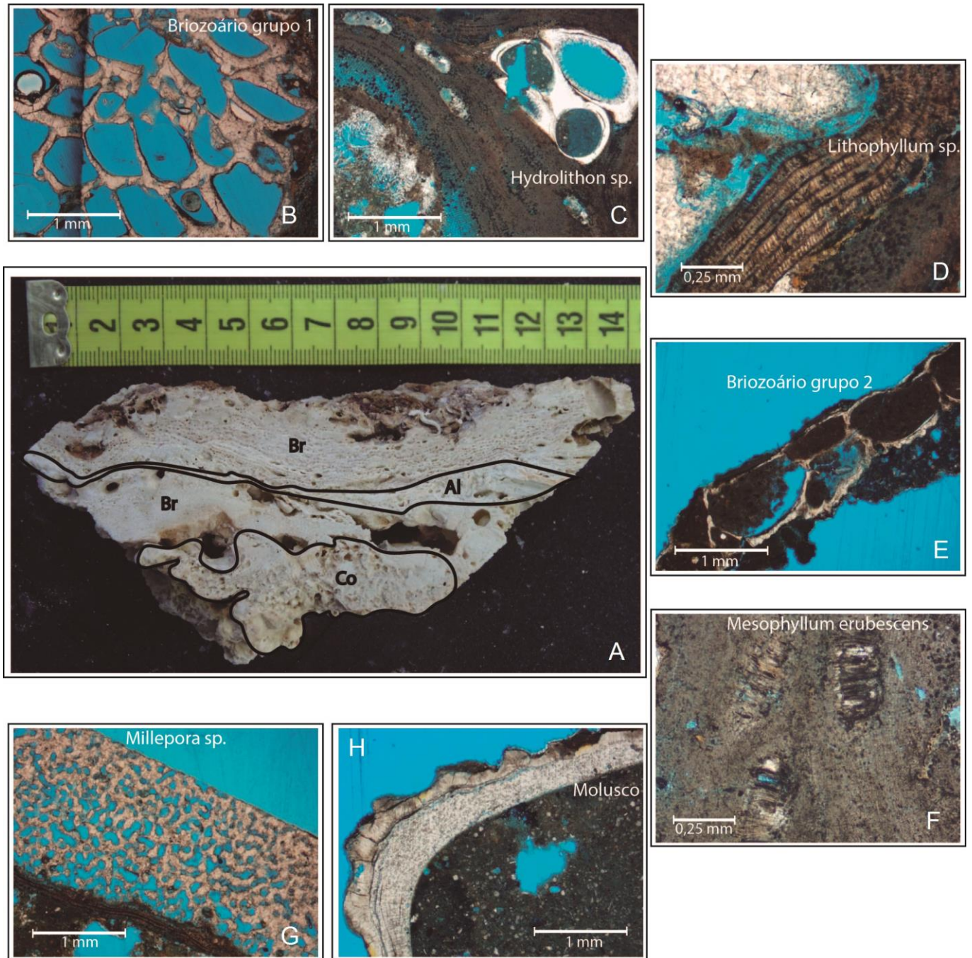
Figura X: Fragmento 8E, localizado próximo ao centro do testemunho horizontal LG-AB-DR 08, e suas respectivas imagens de lâminas petrográficas. (A) Imagem macroscópica do fragmento recifal, onde são evidenciados Alga Calcária (Al), Briozoário (Br) e Coral (Co). (B) Imagem de lâmina microscópica evidenciando Briozoário grupo 1 (C) Imagem de lâmina microscópica evidenciando alga calcária da espécie Hydrolithon sp. (D) Imagem de lâmina microscópica evidenciando alga calcária da espécie Lithophyllum sp. (E) Imagem de lâmina microscópica evidenciando Briozoário grupo 2. (F) Imagem de lâmina microscópica evidenciando alga calcária da espécie Mesophyllum erubescens . (G) Imagem de lâmina microscópica evidenciando coral da espécie Millepora sp. e (H) Imagem de lâmina microscópica evidenciando Molusco.
