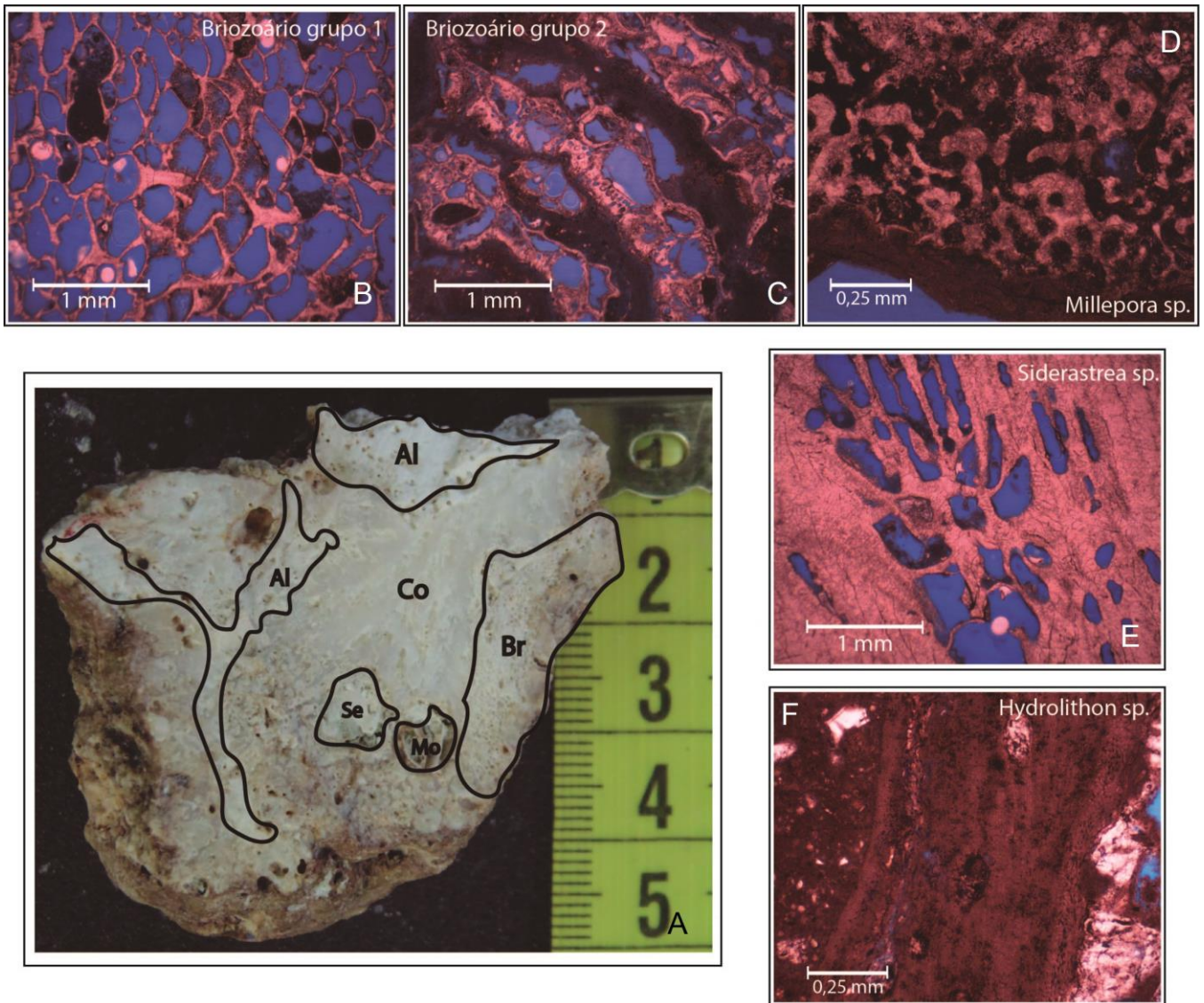
Figura V: Fragmento 6C, localizado próximo ao topo do testemunho vertical LG-AB-DR 06, e suas respectivas imagens de lâminas petrográficas. (A) Imagem macroscópica do fragmento recifal, onde são evidenciados Alga Calcária (Al), Coral (Co), Sedimento fino (Se), Briozoário (Br) e Molusco (Mo). (B) Imagem de lâmina microscópica evidenciando Briozoário grupo 1. (C) Imagem de lâmina microscópica evidenciando Briozoário grupo 2. (D) Imagem de lâmina microscópica evidenciando coral da espécie Millepora sp. (E) Imagem de lâmina microscópica evidenciando coral da espécie Siderastrea sp. e (F) Imagem de lâmina microscópica evidenciando alga calcária da espécie Hydrolithon sp.
