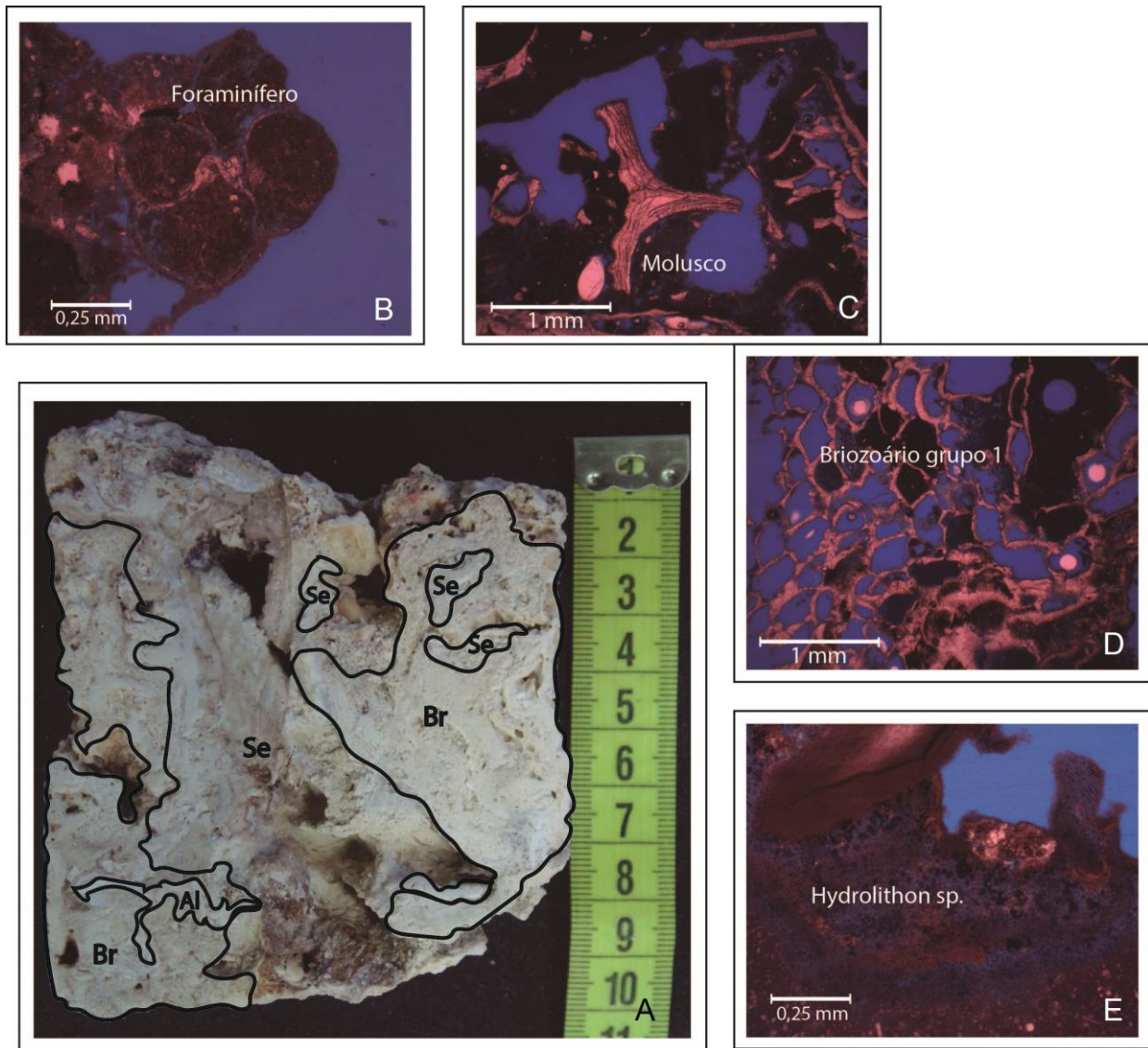
Figura 1: Fragmento 1P, localizado na base do testemunho vertical LG-AB-DR 01, e suas respectivas imagens de lâminas petrográficas. (A) Imagem macroscópica do fragmento recifal, onde são evidenciados Briozoário (Br), Alga Calcária (Al) e Sedimento fino (Se). (B) Imagem de lâmina microscópica evidenciando foraminífero incrustante. (C) Imagem de lâmina microscópica evidenciando fragmento de molusco. (D) Imagem de lâmina microscópica evidenciando briozoário grupo 1 e (E) Imagem de lâmina microscópica evidenciando alga calcária da espécie Hydrolithon sp.
