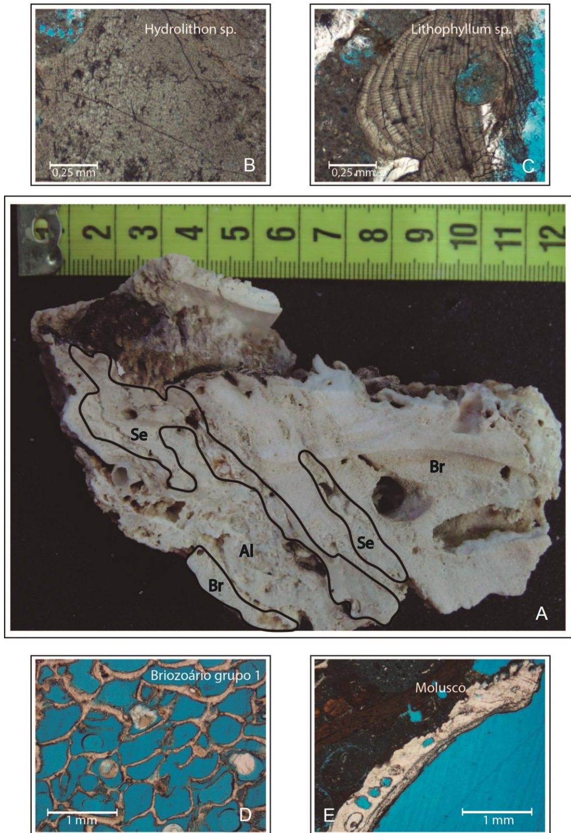
Figura VIII: Fragmento 4E, localizado próximo ao centro do testemunho horizontal LG-AB-DR 04, e suas respectivas imagens de lâminas petrográficas. (A) Imagem macroscópica do fragmento recifal, onde são evidenciados Alga Calcária (Al), Briozóário (Br) e Sedimento fino (Se). (B) Imagem de lâmina microscópica evidenciando alga calcária da espécie Hydrolithon
