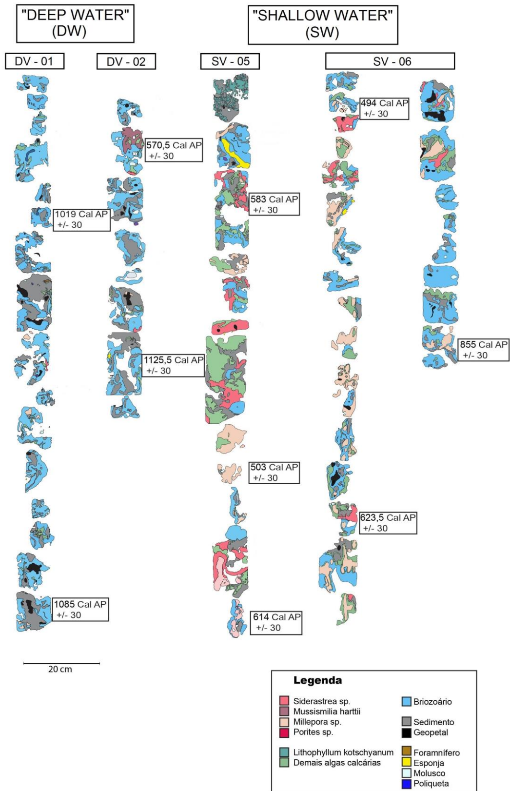
Figura 5: Assembleia dos organismos encontrados nos testemunhos verticais dos ambientes Shallow Water (SW) e Deep Water (DW). Testemunhos DV - 01, DV - 02, SV - 05 e SV - 06. O testemunho SV - 06 foi dividido em duas parcelas para melhor visualização da imagem. Em
