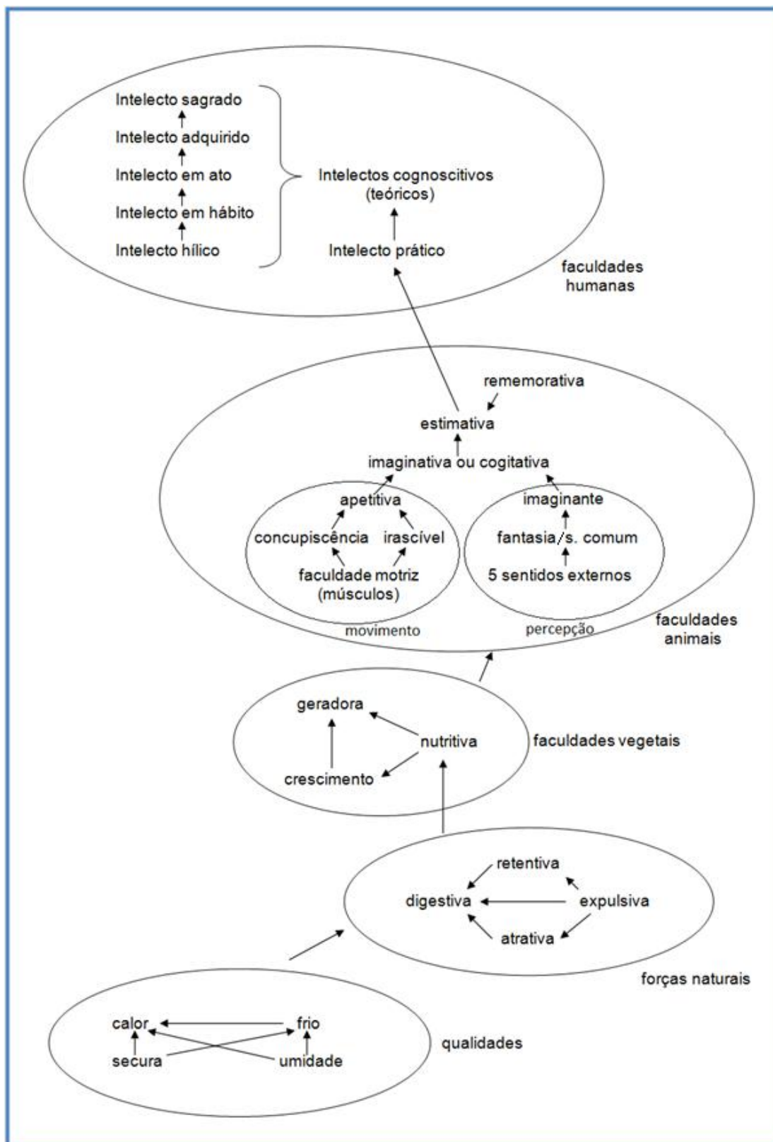
Imagem 05: A partir da descrição feita pelo filósofo nos parágrafos anteriores, compusemos graficamente o esquema hierárquico das faculdades humanas, animais e vegetais, bem como das forças naturais e qualidades. A direção das setas indica qual faculdade, força ou qualidade serve a qual.
