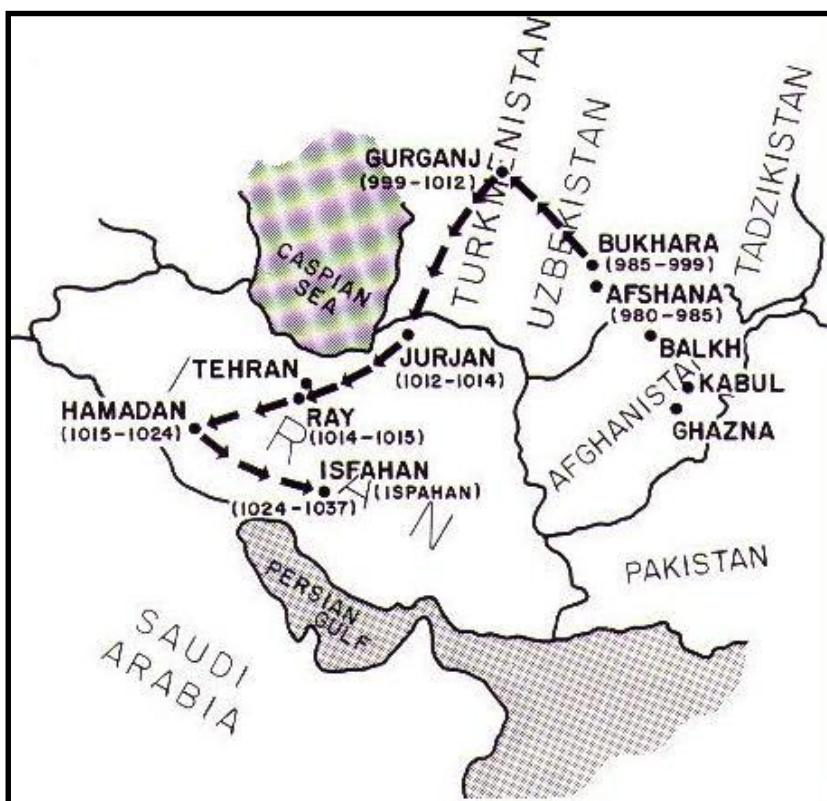
Imagem 01: Esboço de mapa com o itinerário da vida de Ibn Sīnā e datas aproximadas das fases de sua vida. Notar, no capítulo em diante, os motivos pelos quais discordamos das datas propostas
