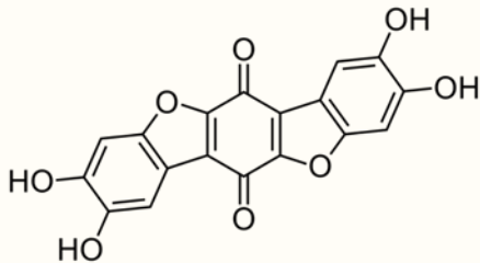
Ácido telefórico
