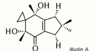
illudin A
