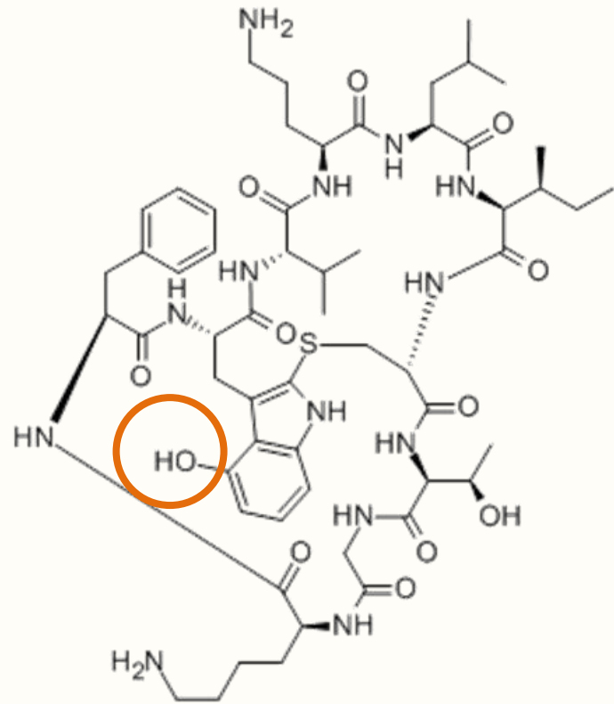
Cortinarina B
