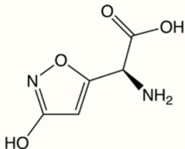
Ácido iboténico
