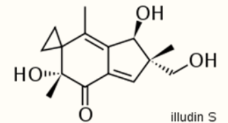
illudin S
