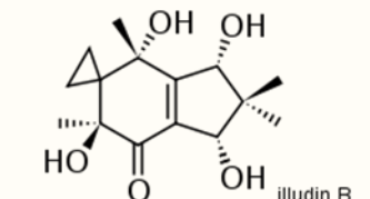
illudin B
