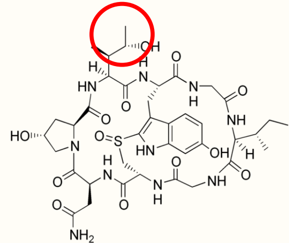
Amanitina \gamma
