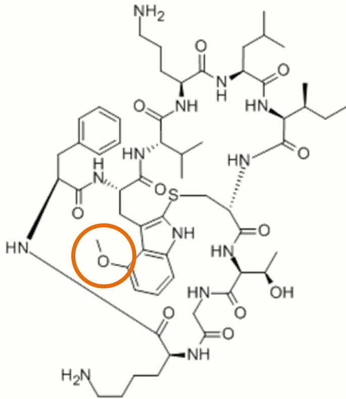
Cortinarina A
