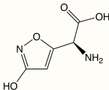
Muscazóna
