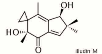
illudin M
