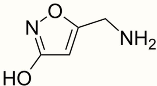
Muscimol
