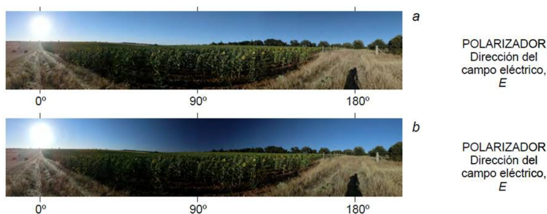
Figura 5. Fotografías panorámicas de 180^\circ con el Sol próximo a la línea del horizonte, tomadas con filtro polarizador. (a) Con dirección de polarización del campo eléctrico vertical. (b) Con dirección de polarización del campo eléctrico horizontal. En este caso el cielo se observa más oscuro a 90^\circ del Sol.
